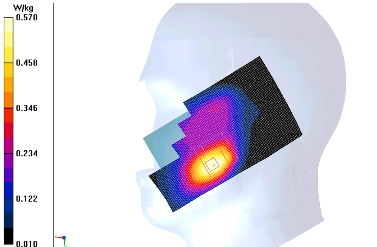
Fig.7 WCDMA1900 CH9400
