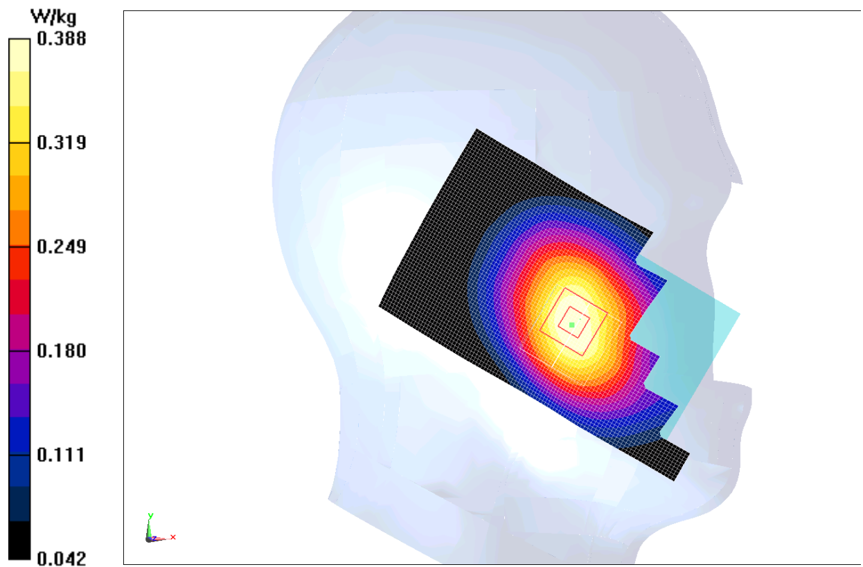
Fig.J.1 850MHz CH190
