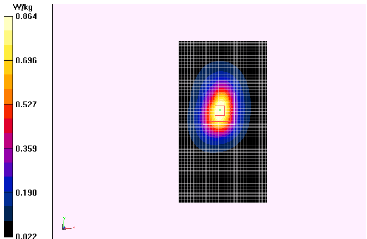
Fig.J.4 GSM 1900MHz CH810
