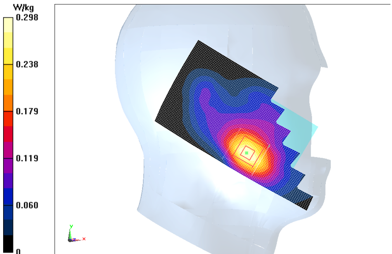
Fig.J.3 GSM 1900MHz CH661
