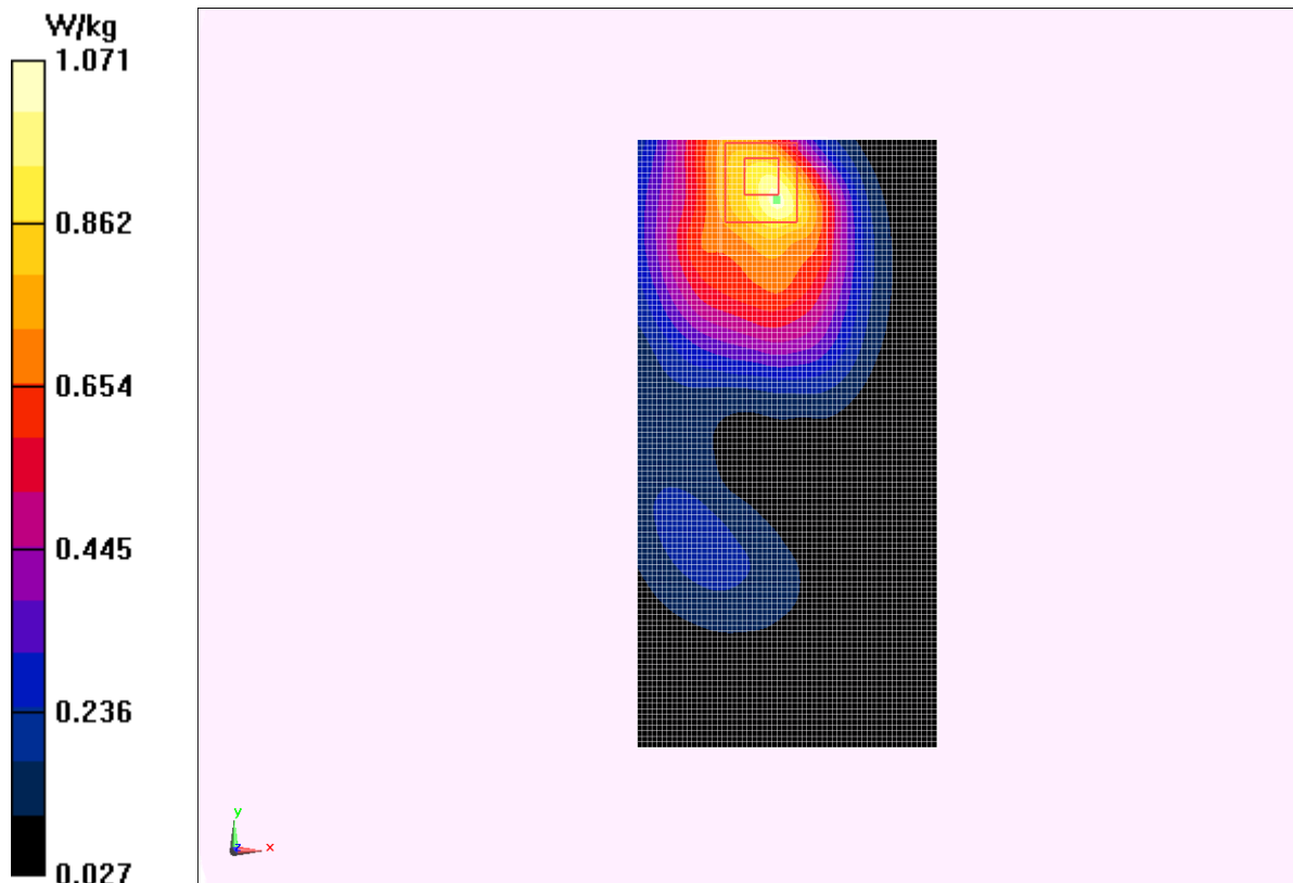
Fig.8 WCDMA1900 CH9400
