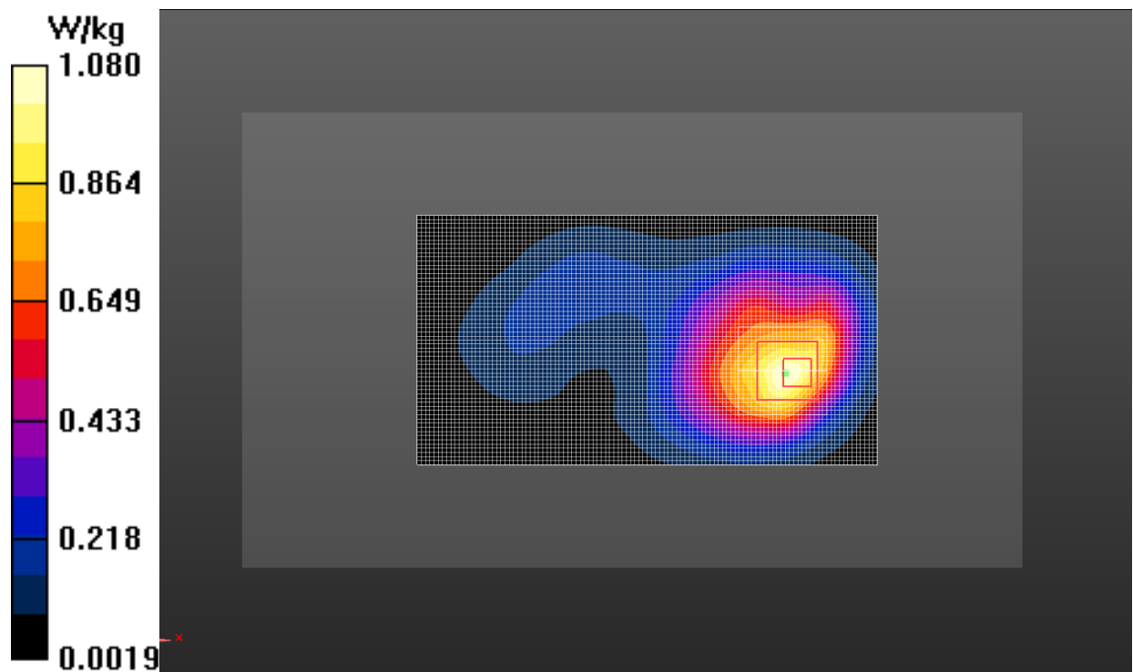
Fig.8 WCDMA1900 CH9400
