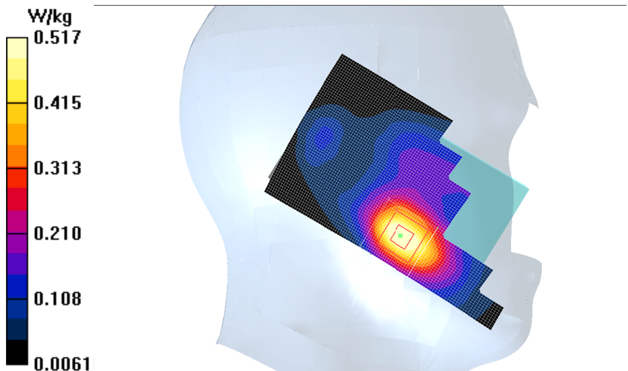
Fig.7 WCDMA1900 CH9538
