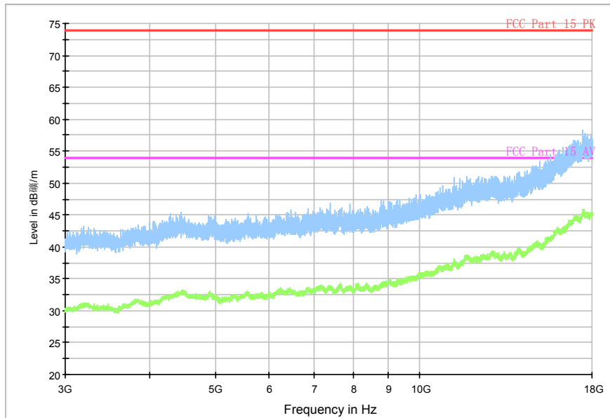
RE - 3GHz-18GHz
