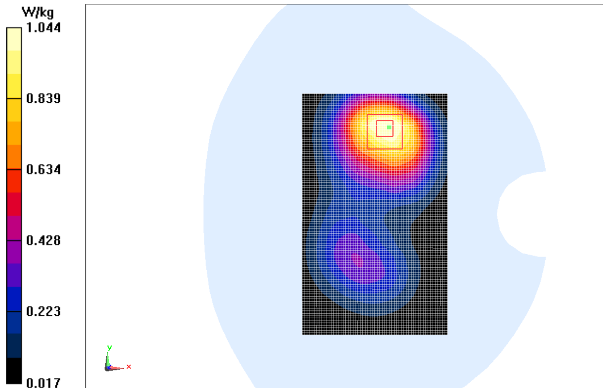
Fig.8 WCDMA1900 CH9262
