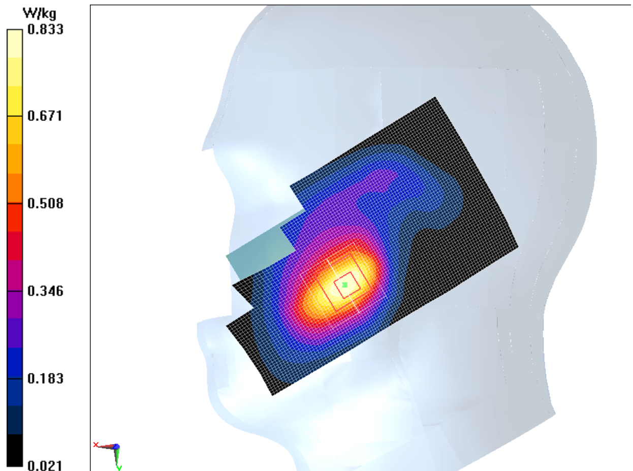
Fig.7 WCDMA1900 CH9400
