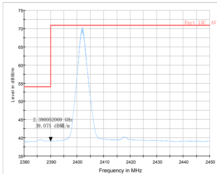
RE - Power-2.38GHz-2.45GHz-BT AV
