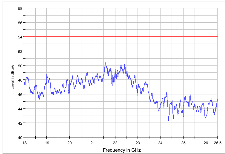
EMI 18GHz-26.5GHz
