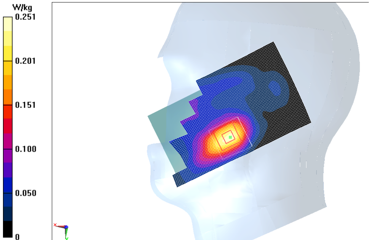
Fig.7 WCDMA1900 CH9400
