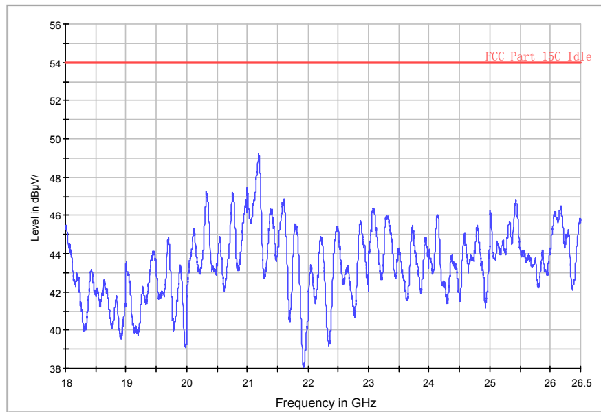
EMI 18GHz-26.5GHz
