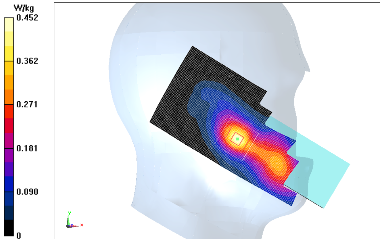
Fig.7 WCDMA1900 CH9538
