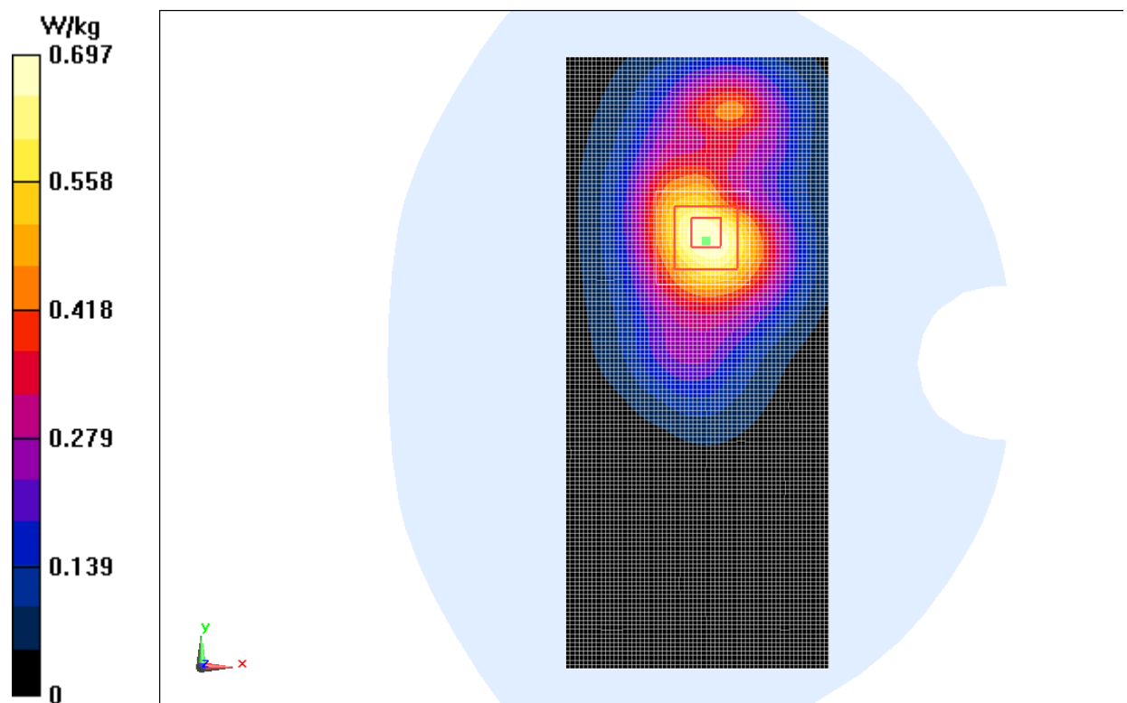
Fig.8 WCDMA1900 CH9262
