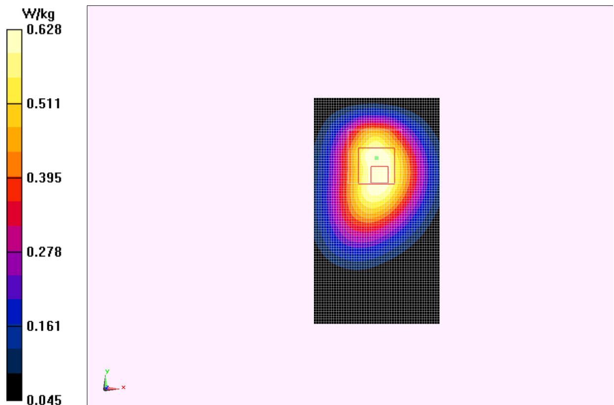
Fig. A.2 850 MHz CH128
