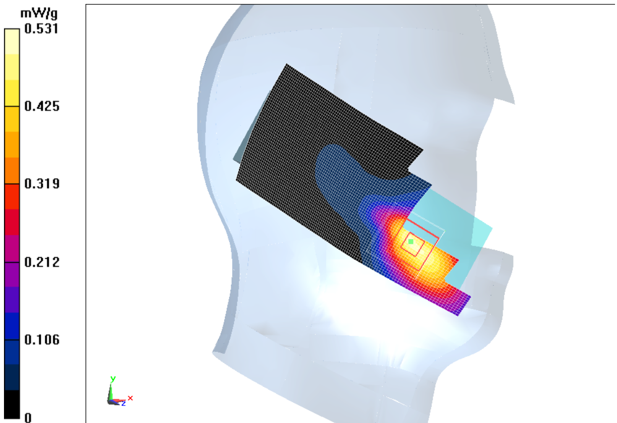
Fig. A.3 1900 MHz CH810
