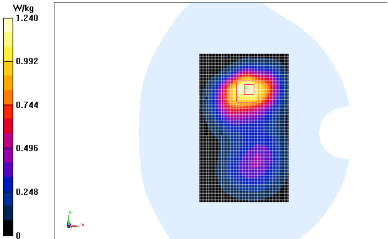
Fig.8 WCDMA1900 CH9262
