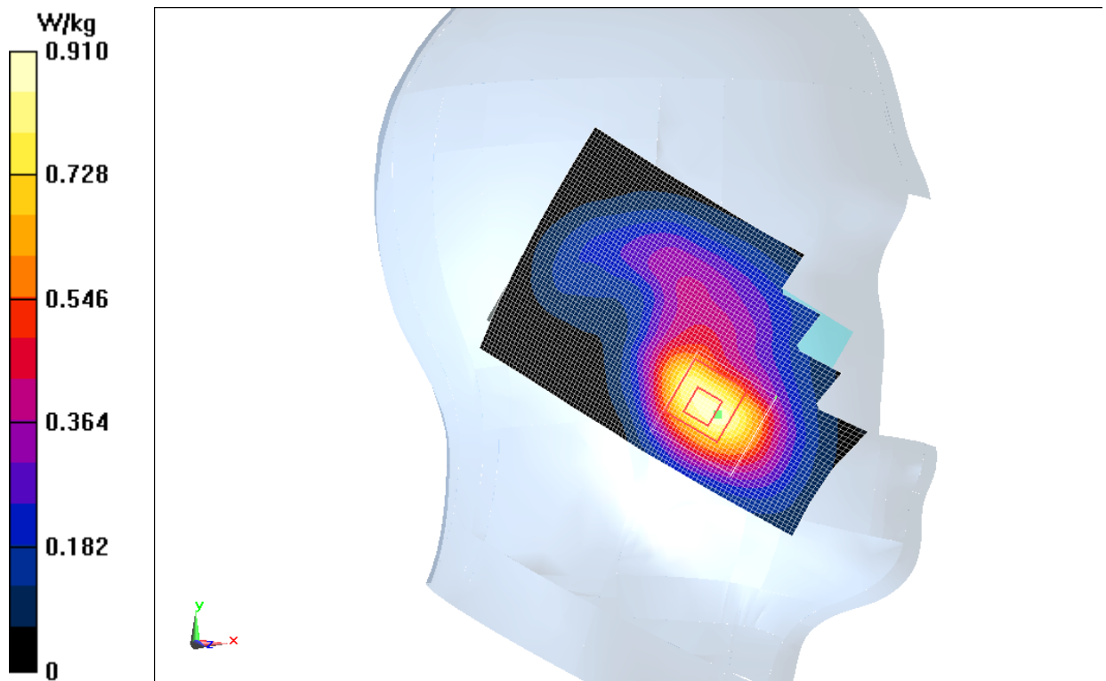
Fig.7 WCDMA1900 CH9538
