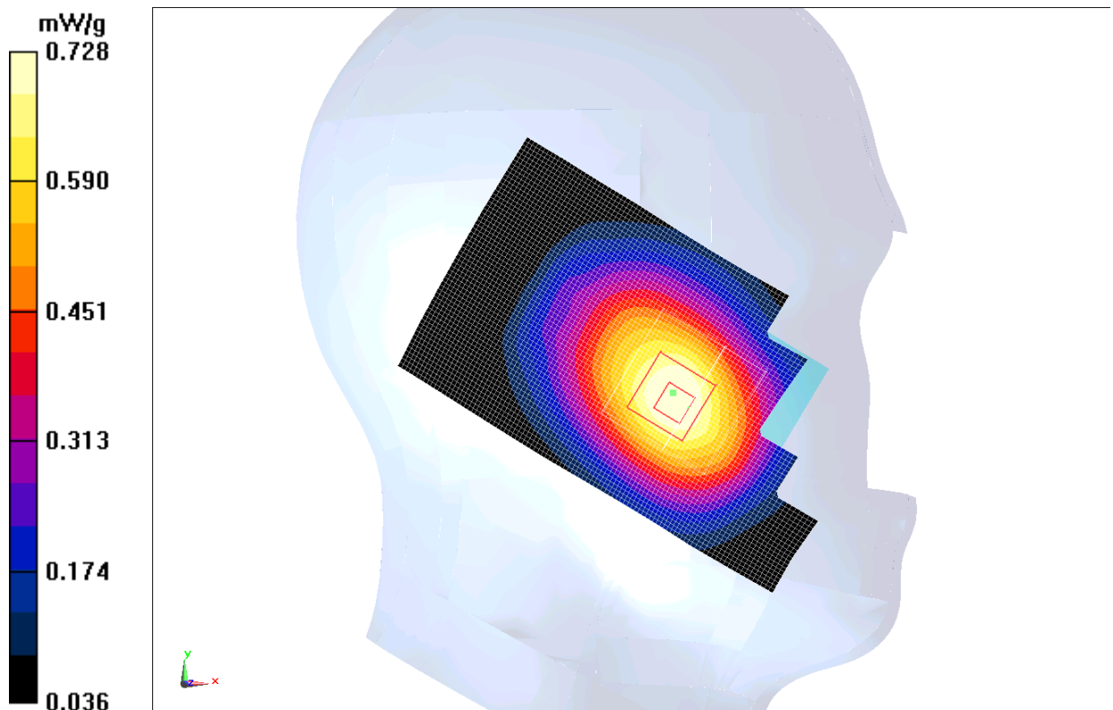
Fig. 1 850MHz CH251
