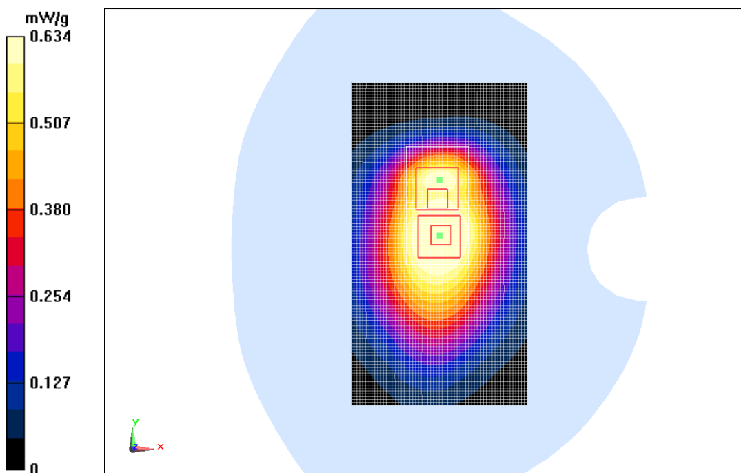
Fig. 22 850 MHz CH251
