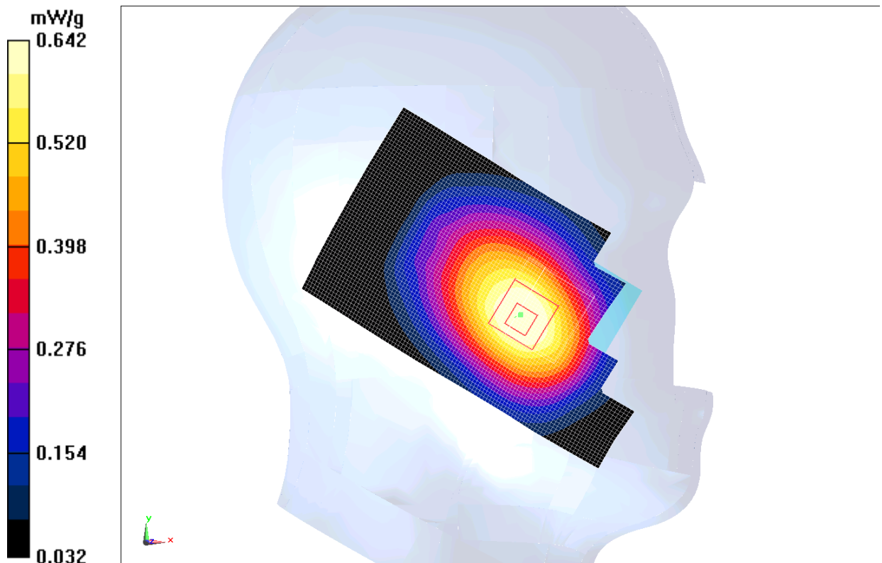
Fig. 2 850 MHz CH190
