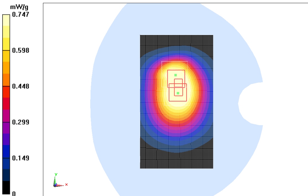
Fig. 21 850 MHz CH251
