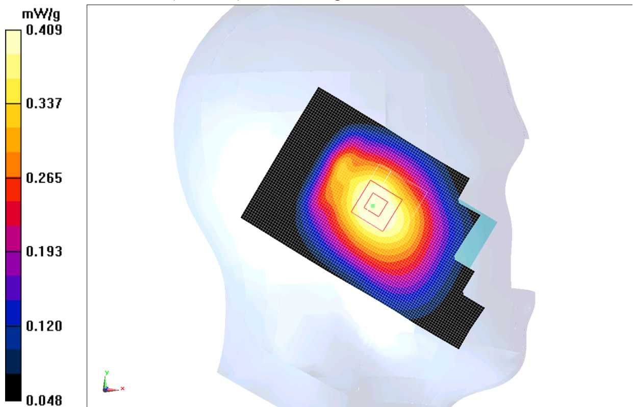
Fig. 6 850 MHz CH128
