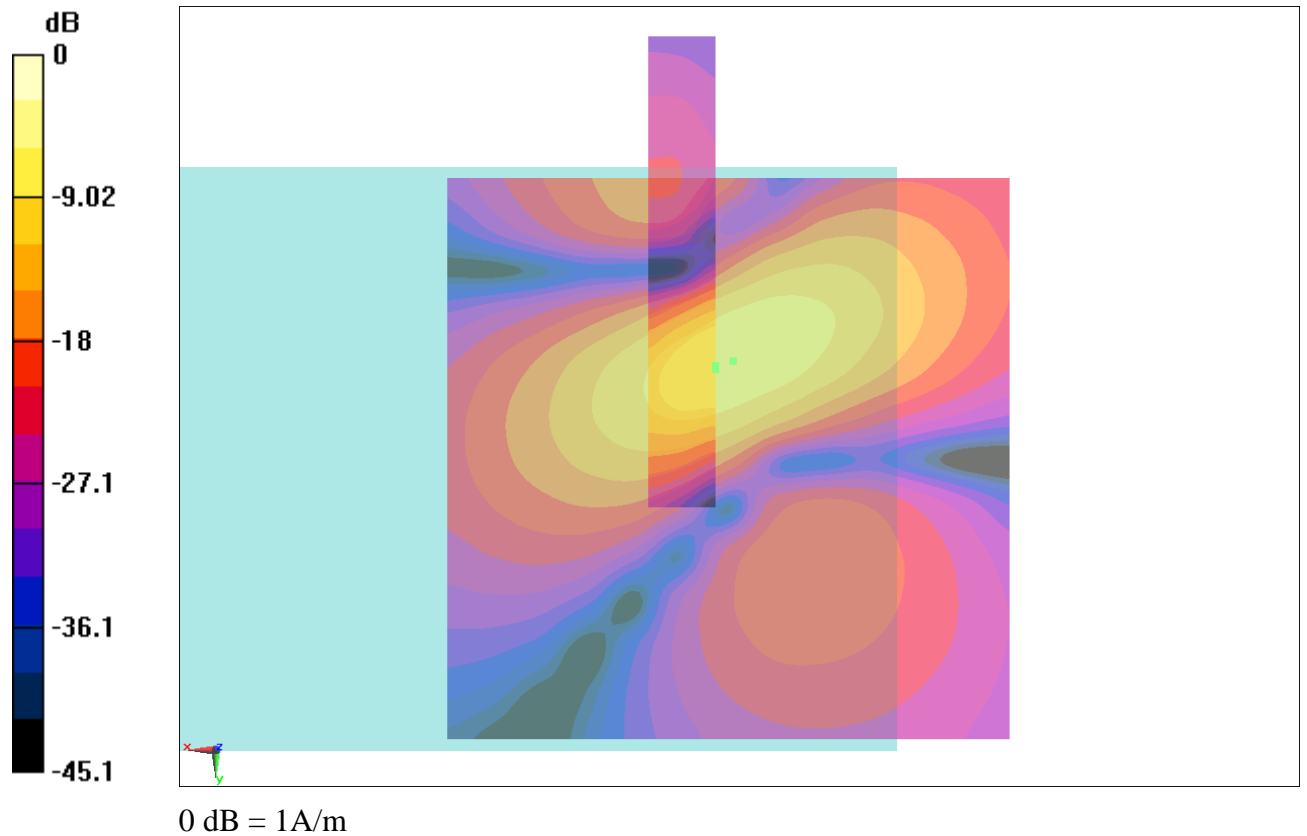
Fig B.11 T-Coil WCDMA 1700
