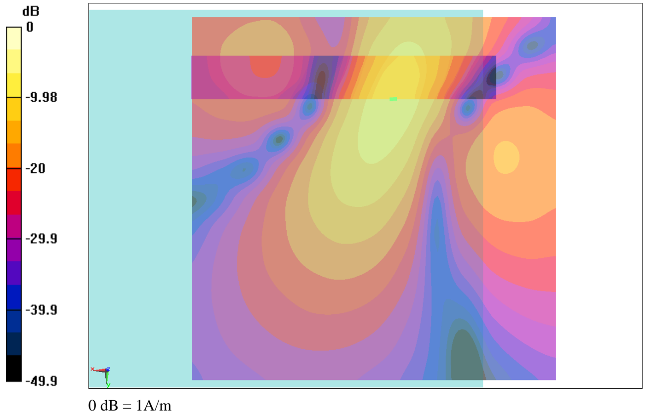
Fig B.7 T-Coil WCDMA 850
