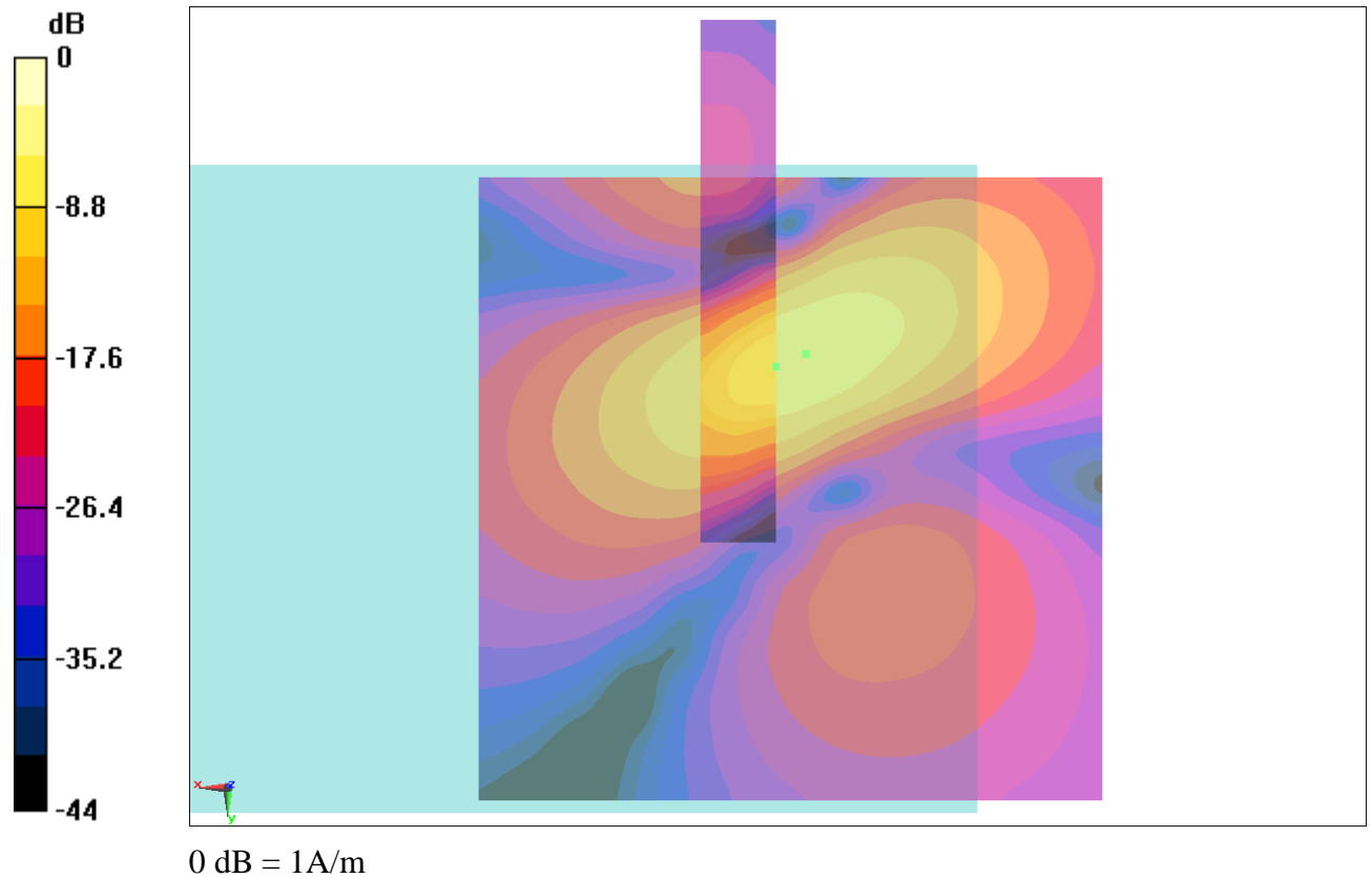
Fig B.8 T-Coil WCDMA 850
