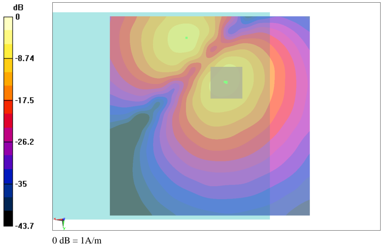
Fig B.3 T-Coil GSM 850
