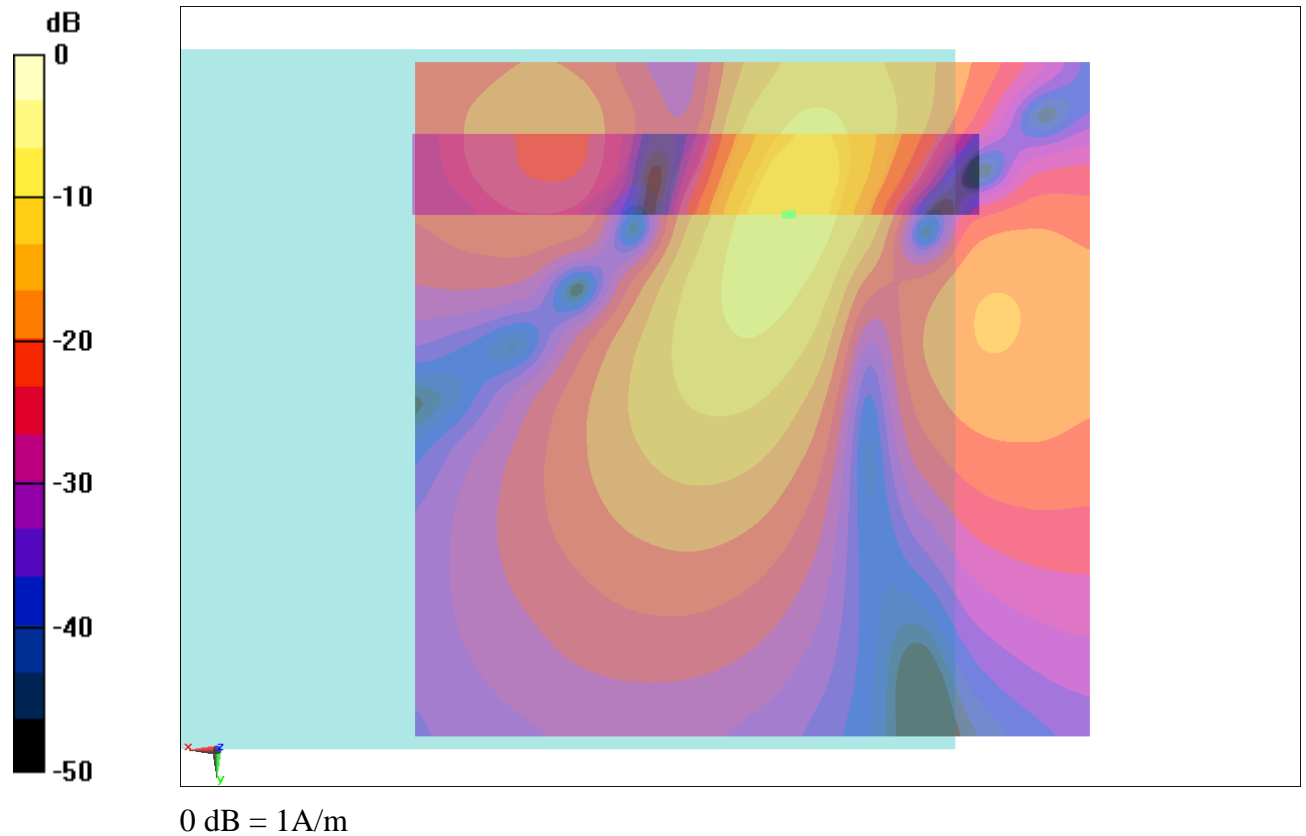
Fig B.13 T-Coil WCDMA 1900
