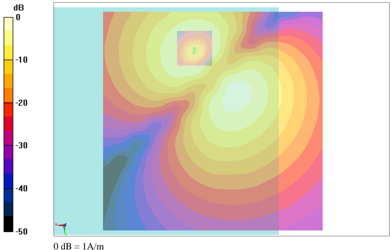
Fig B.12 T-Coil WCDMA 1700
