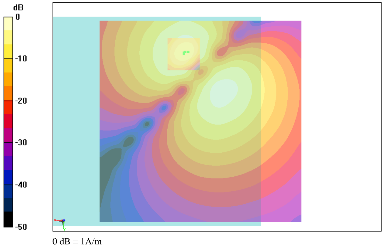
Fig B.15 T-Coil WCDMA 1900
