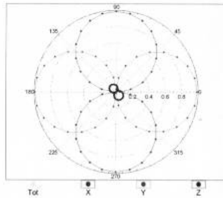
f=2500 MHz,R22,0°
