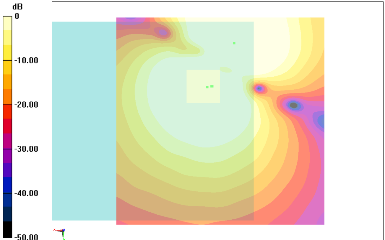
Fig B.3 T-Coil GSM 850
