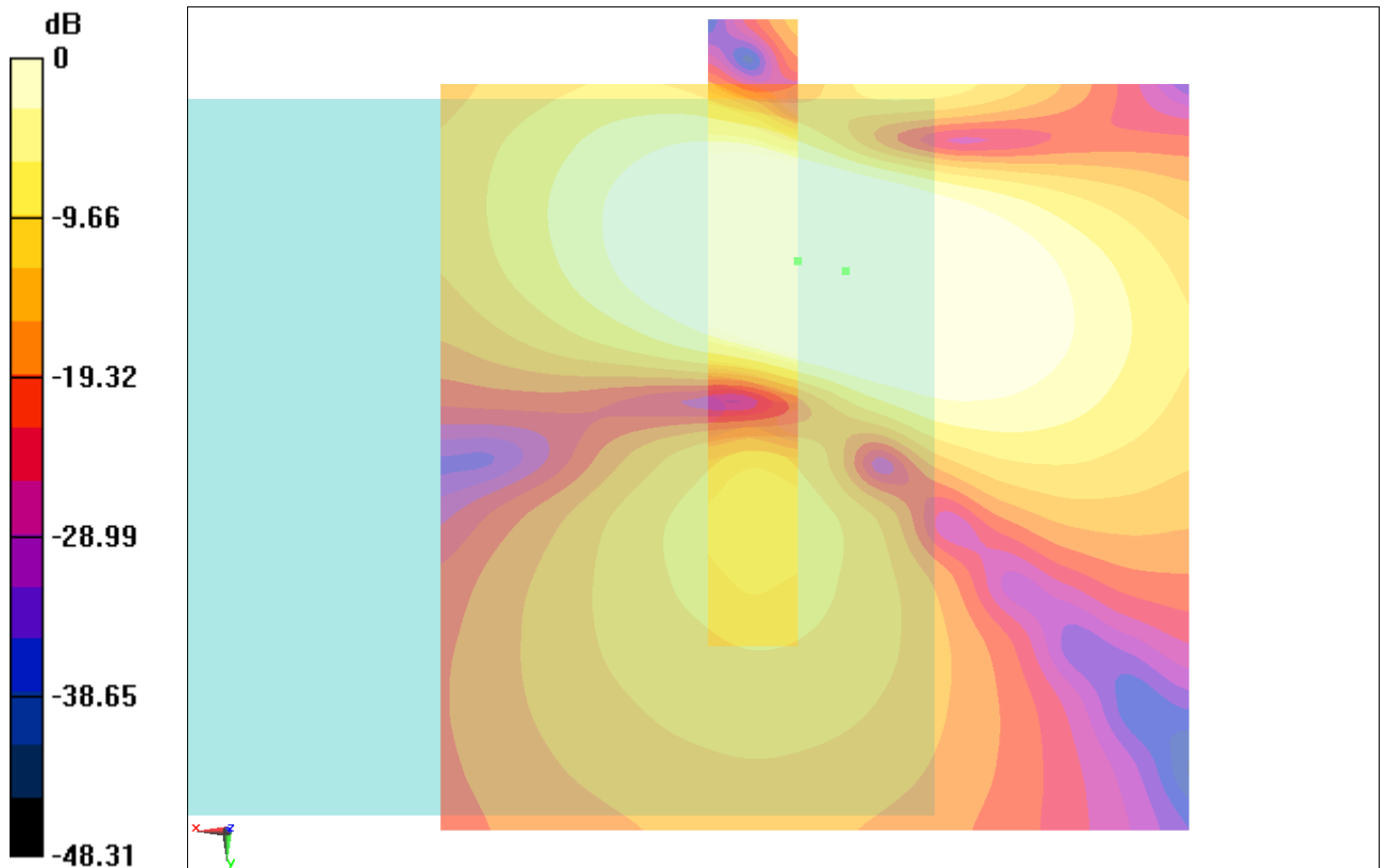
Fig B.11 T-Coil WCDMA 1900
