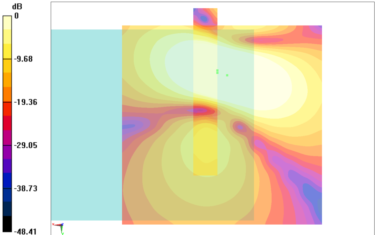
Fig B.8 T-Coil WCDMA 850
