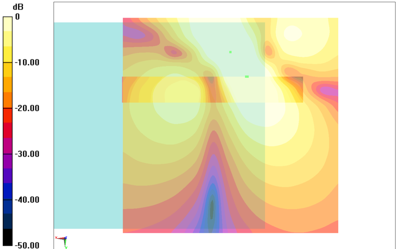
Fig B.7 T-Coil WCDMA 850
