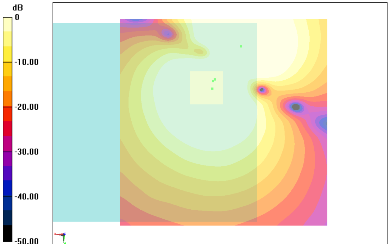
Fig B.9 T-Coil WCDMA 850
