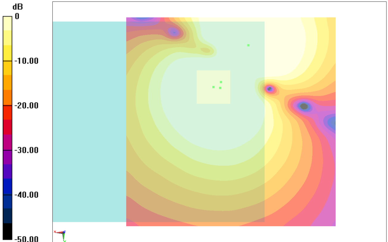
Fig B.12 T-Coil WCDMA 1900
