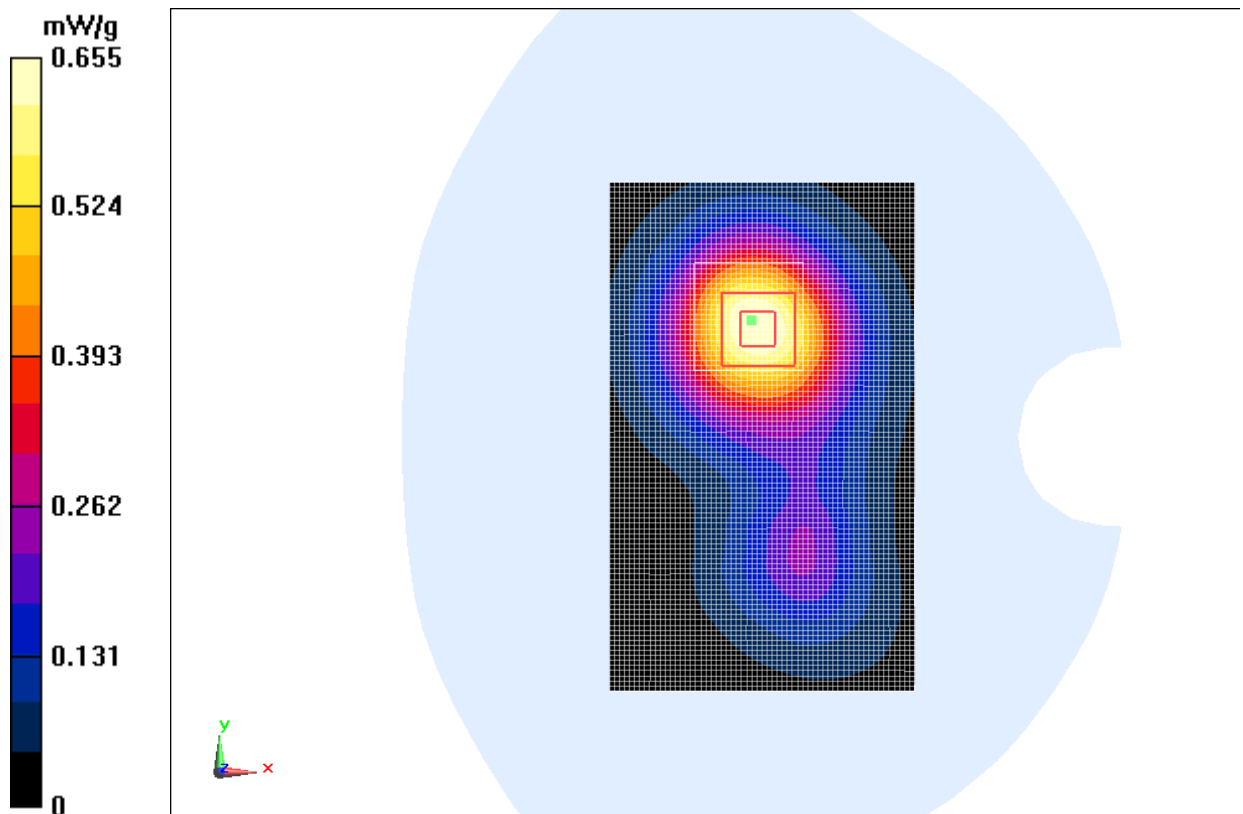
Fig. 82 WCDMA1900 CH9262
