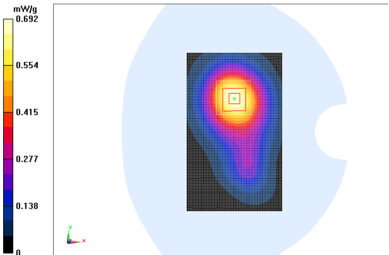
Fig. 81 WCDMA1900 CH9400
