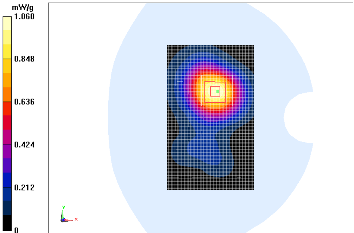
Fig. 83 WCDMA1900 CH9400
