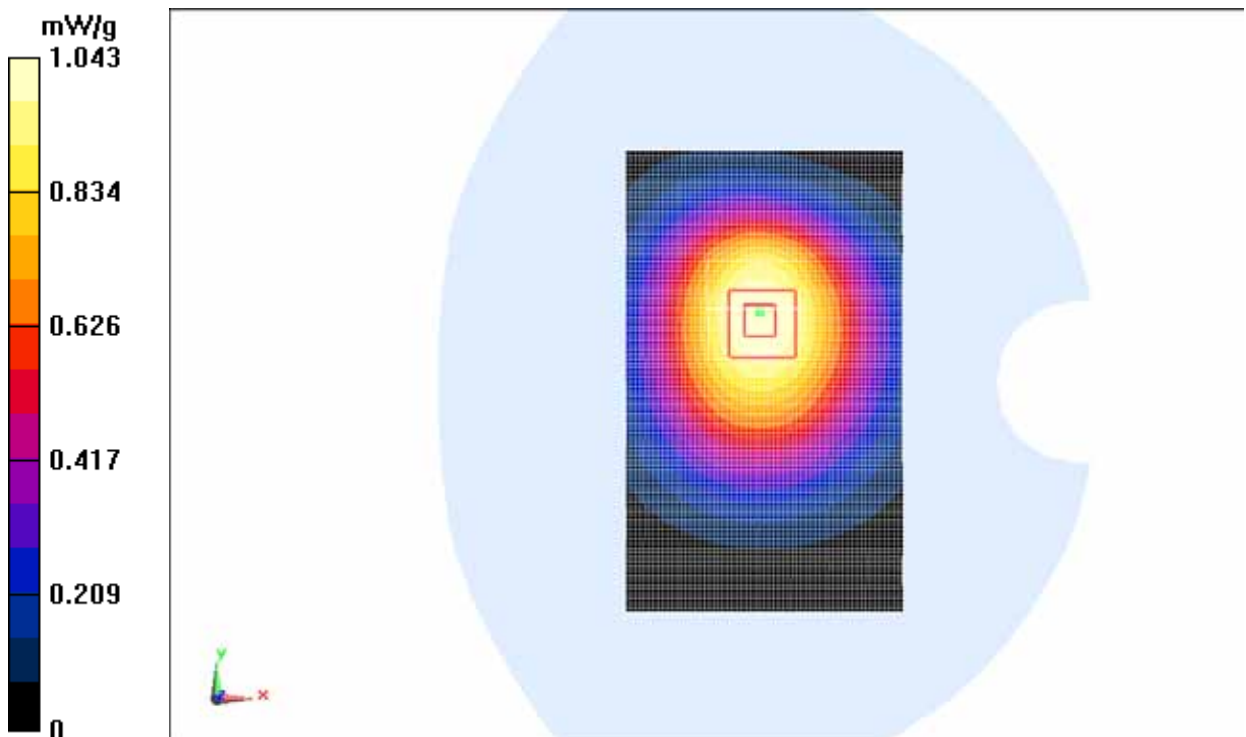
Fig. 13 850 MHz CH251
