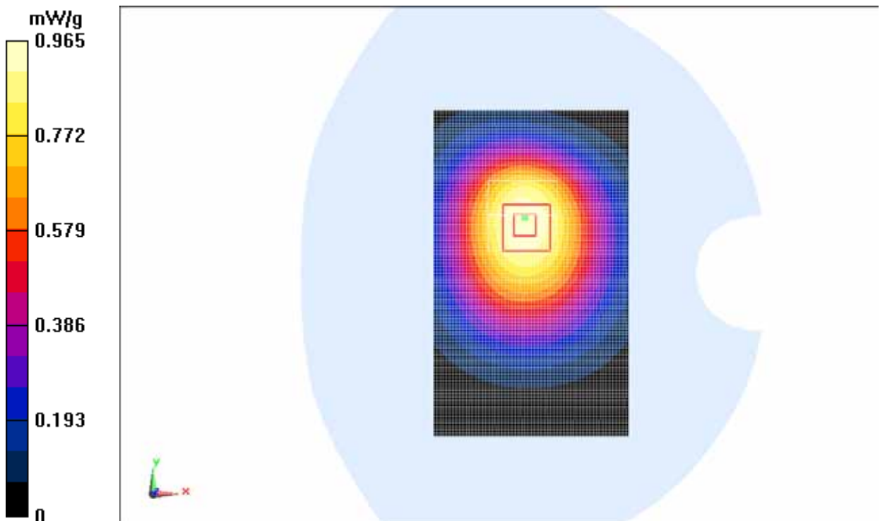
Fig. 14 850 MHz CH190
