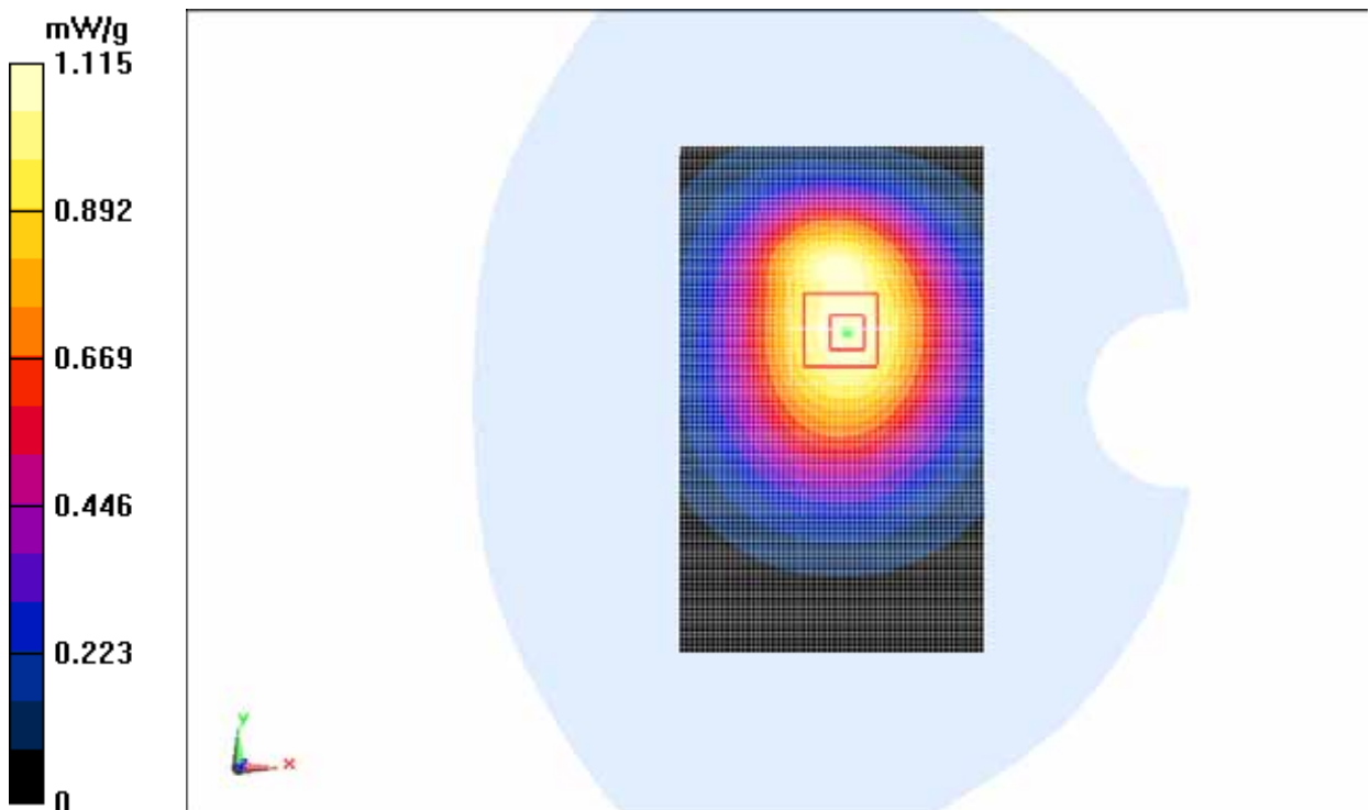
Fig. 16 850 MHz CH251
