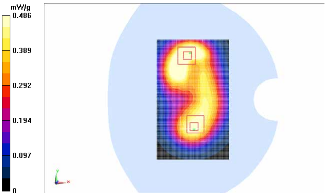
Fig. 33 1900 MHz CH810
