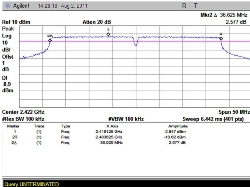
(Plot A: Channel 3: 2422MHz)
