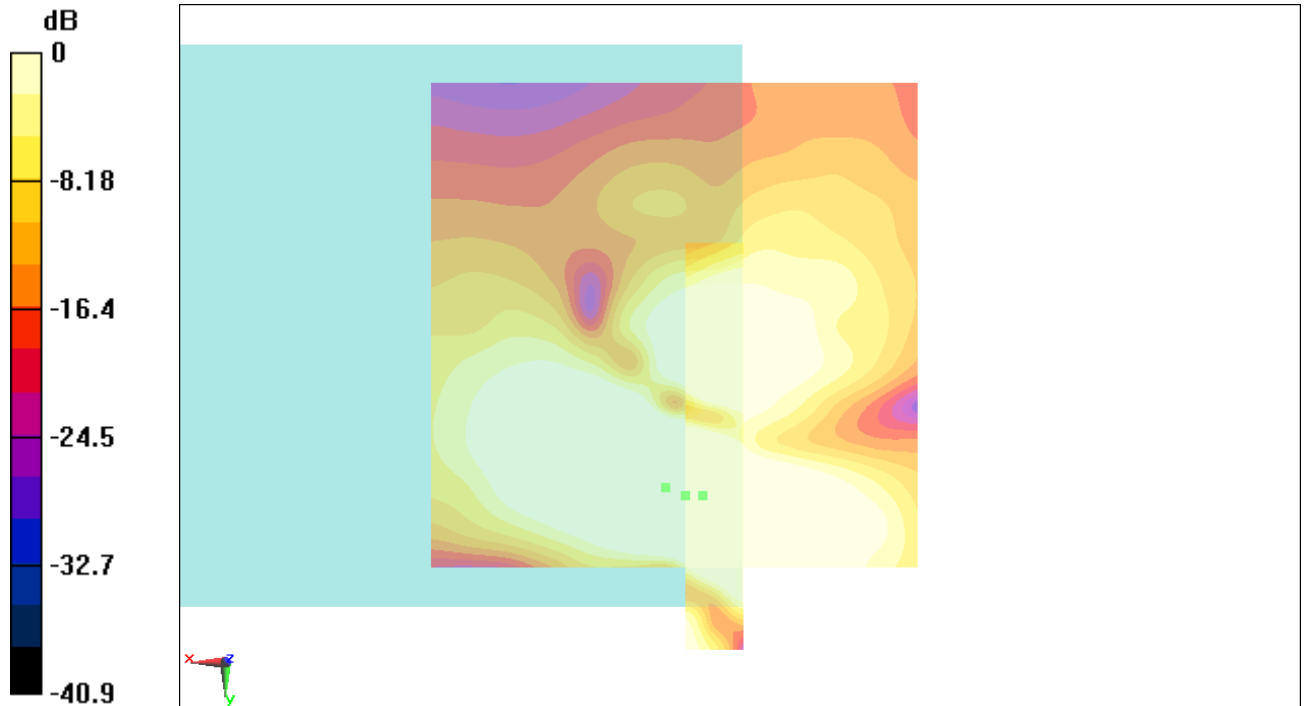
Fig B.8 T-Coil WCDMA 850
