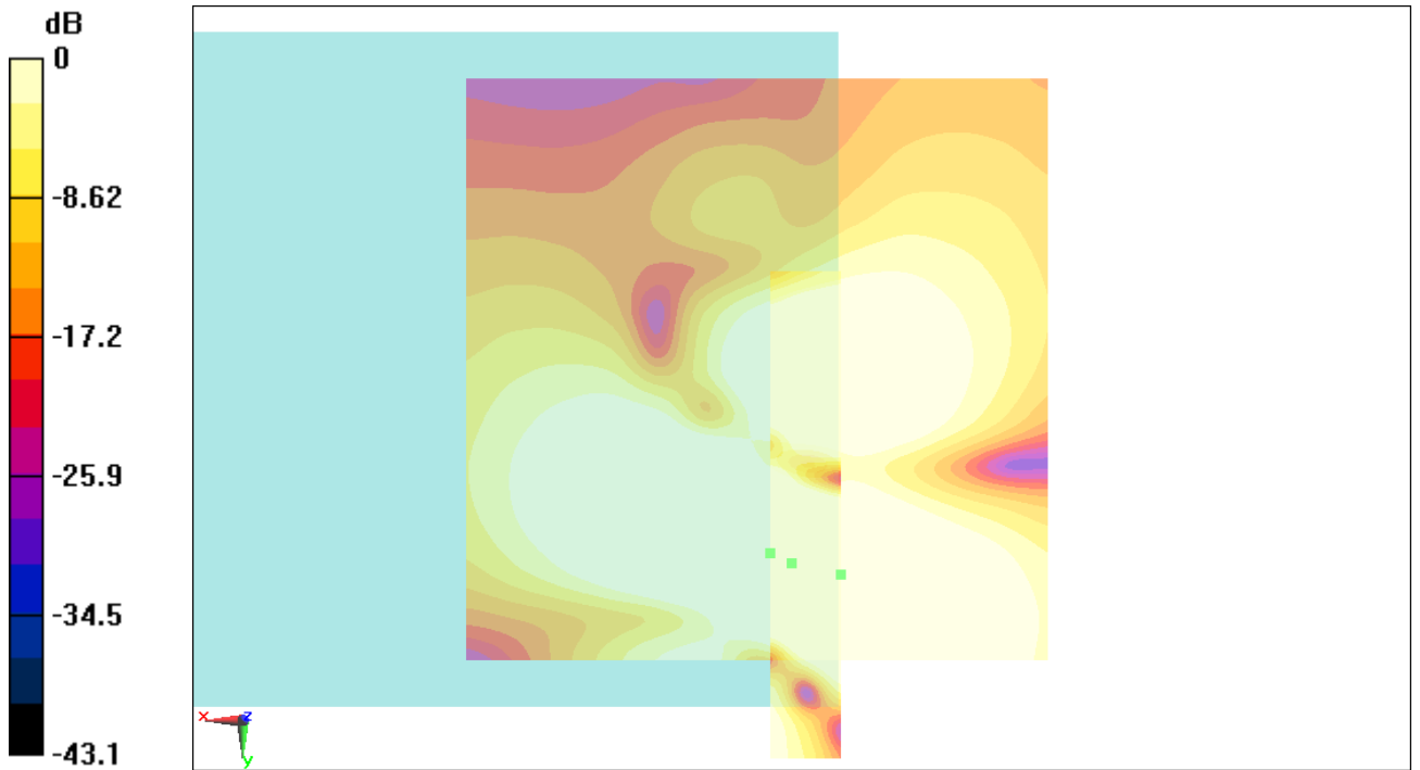
Fig B.11 T-Coil WCDMA 1900
