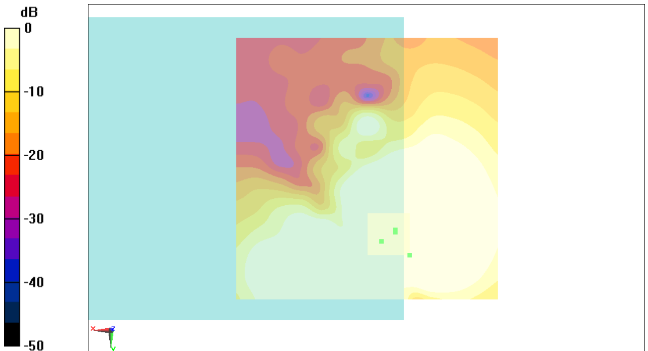
Fig B.12 T-Coil WCDMA 1900
