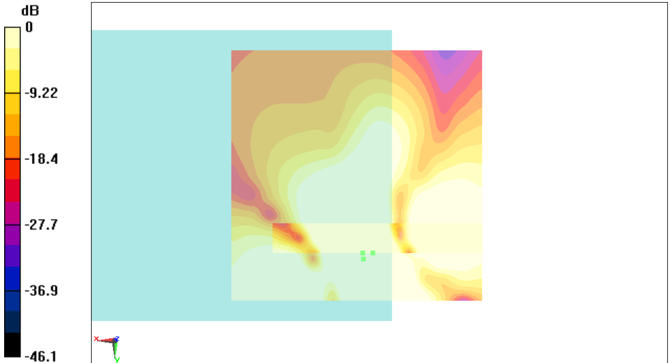
Fig B.7 T-Coil WCDMA 850
