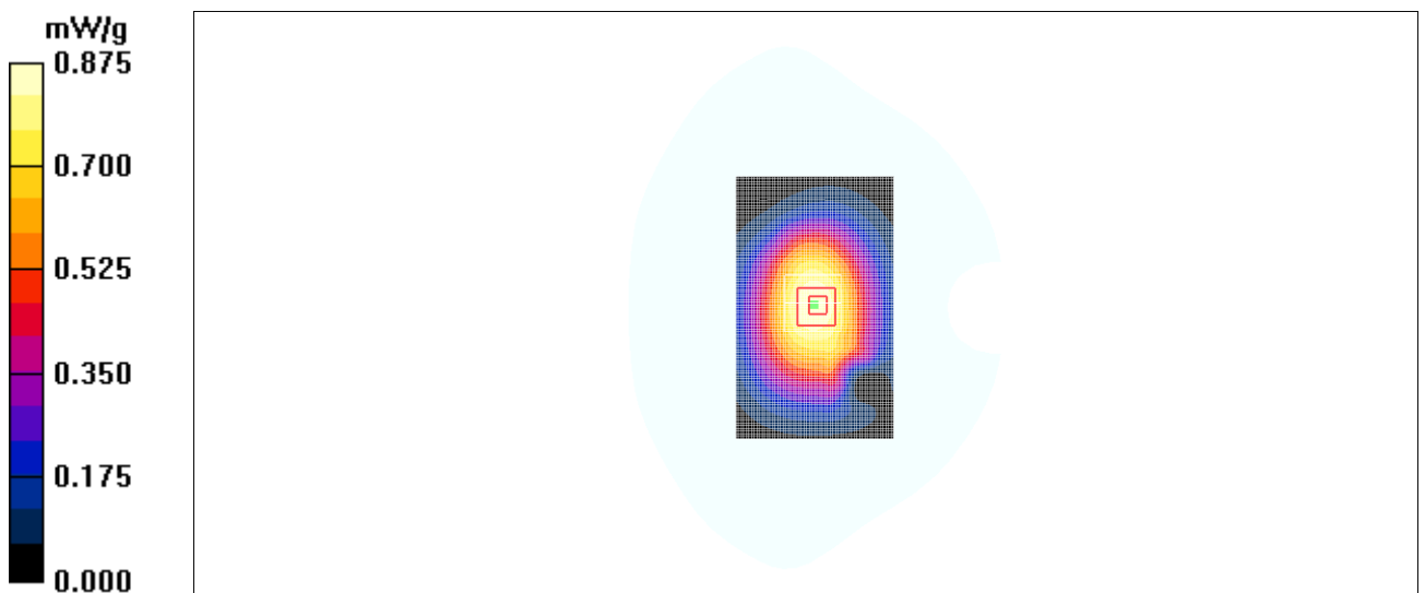
Fig. 50 850 MHz CH190
