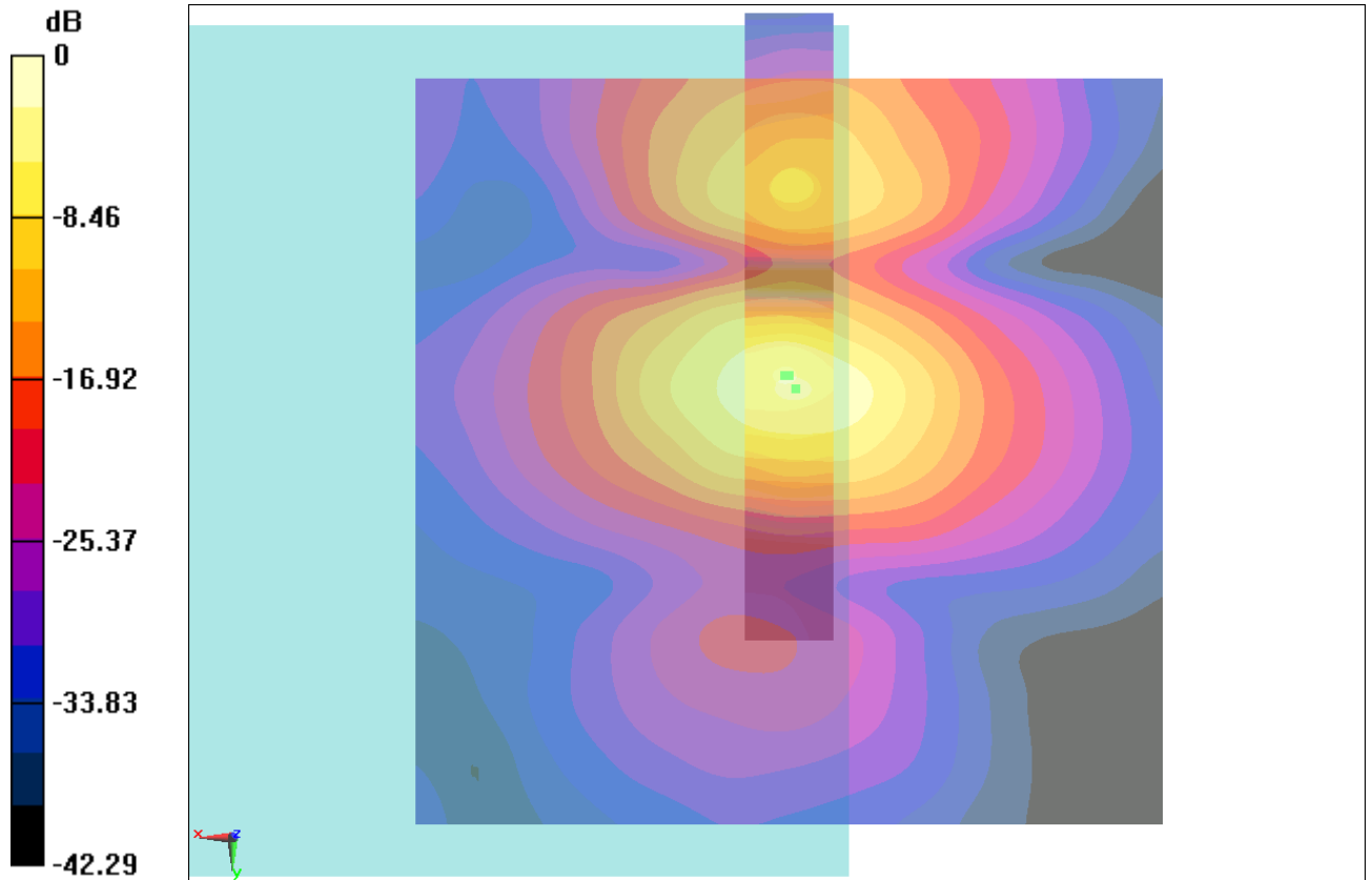
Fig B.5 T-Coil CDMA 835_Channel 384
