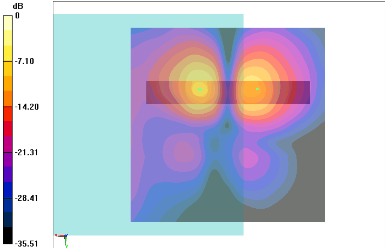
Fig B.4 T-Coil CDMA 835_Channel 384
