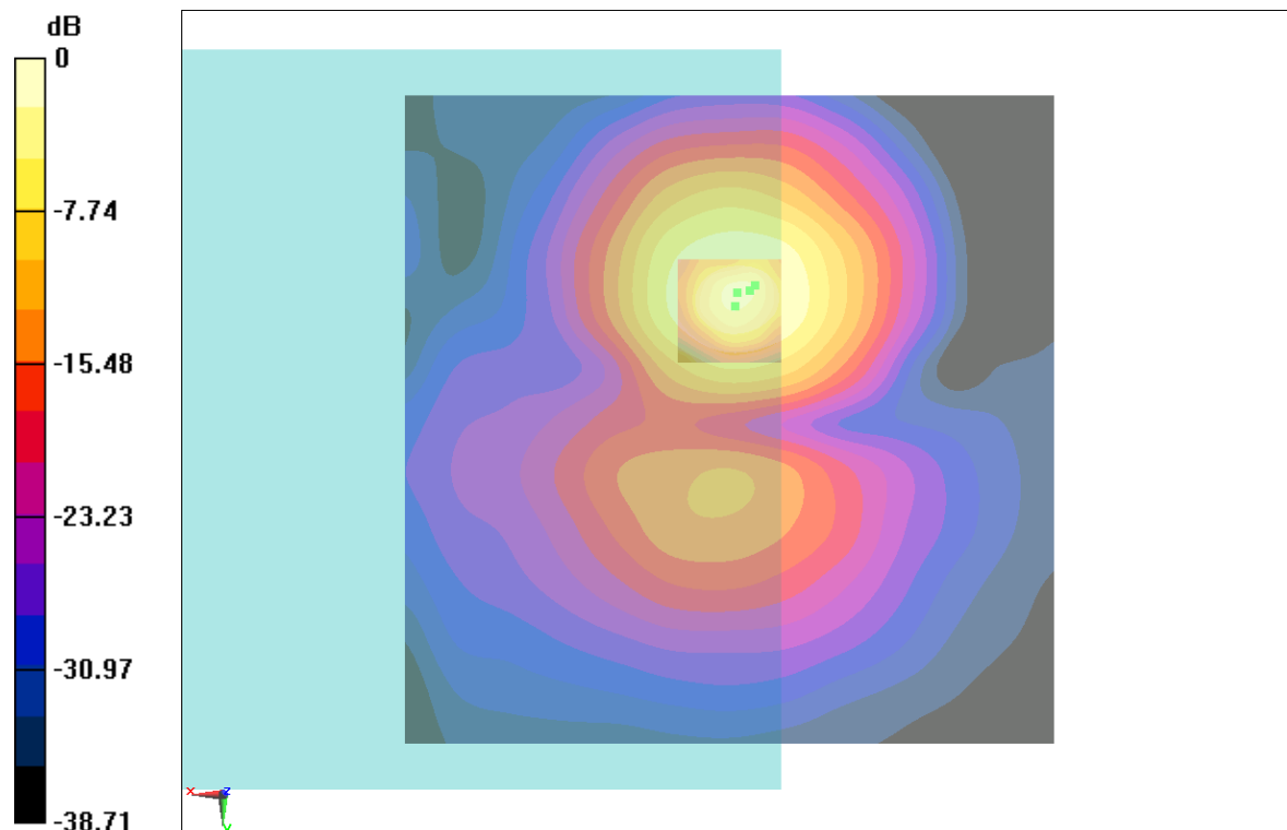
Fig B.6 T-Coil CDMA 835_Channel 384
