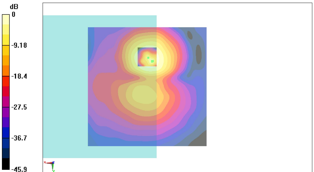
Fig B.6 T-Coil CDMA 835_Channel 384
