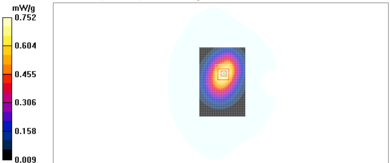
Fig. 47 850 MHz CH251
