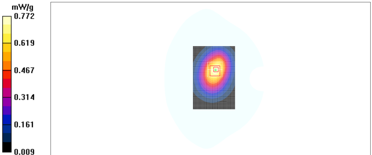
Fig. 45 850 MHz CH251
