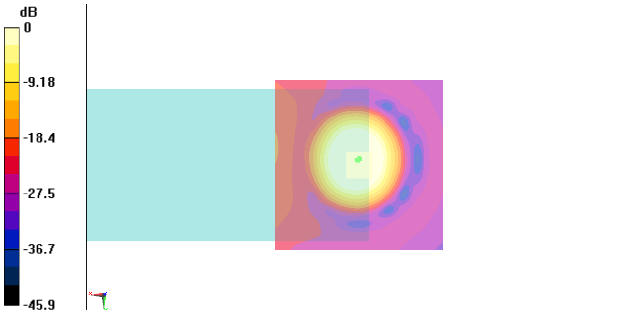
Fig B.3 T-Coil GSM 850
