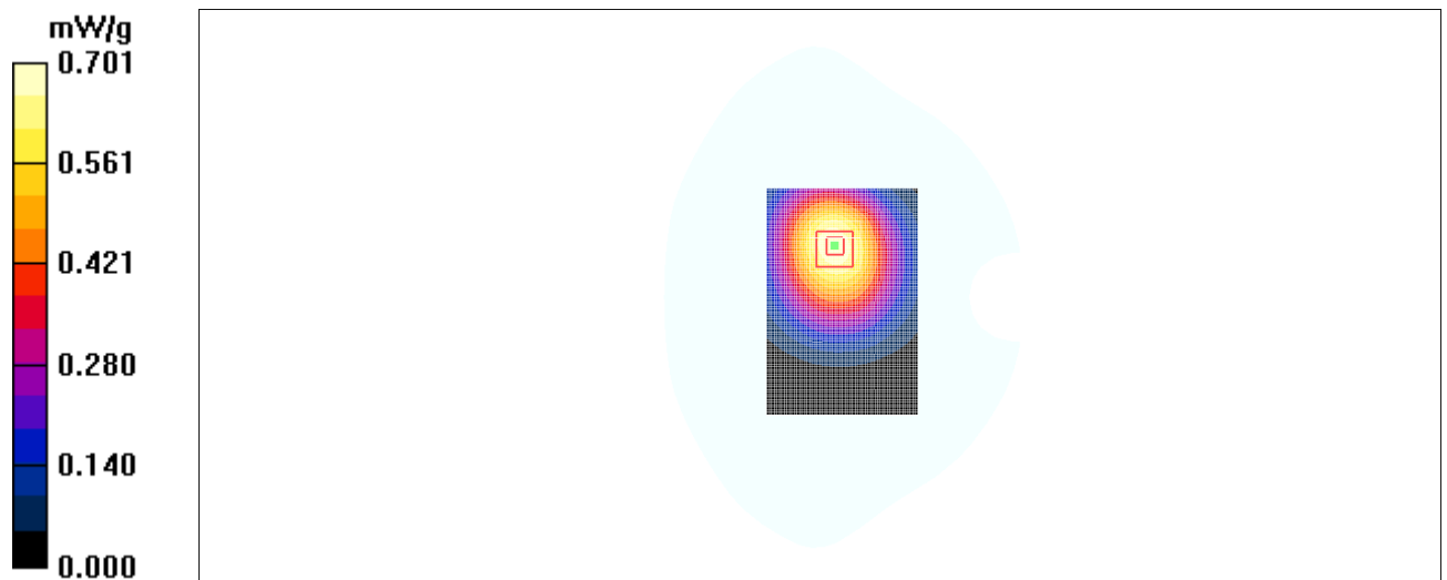
Fig. 28 850 MHz CH251
