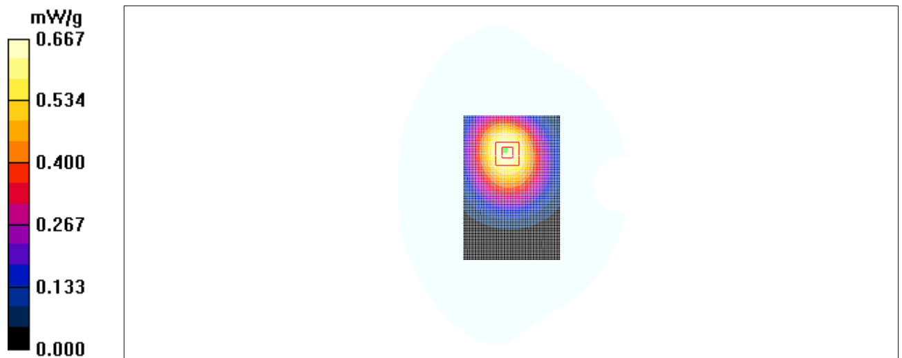
Fig. 29 850 MHz CH190
