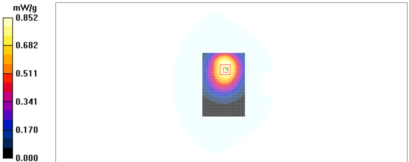
Fig. 26 850 MHz CH190
