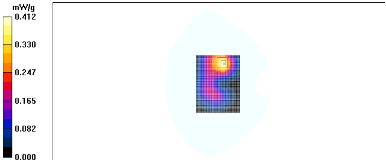
Fig. 33 1900 MHz CH810
