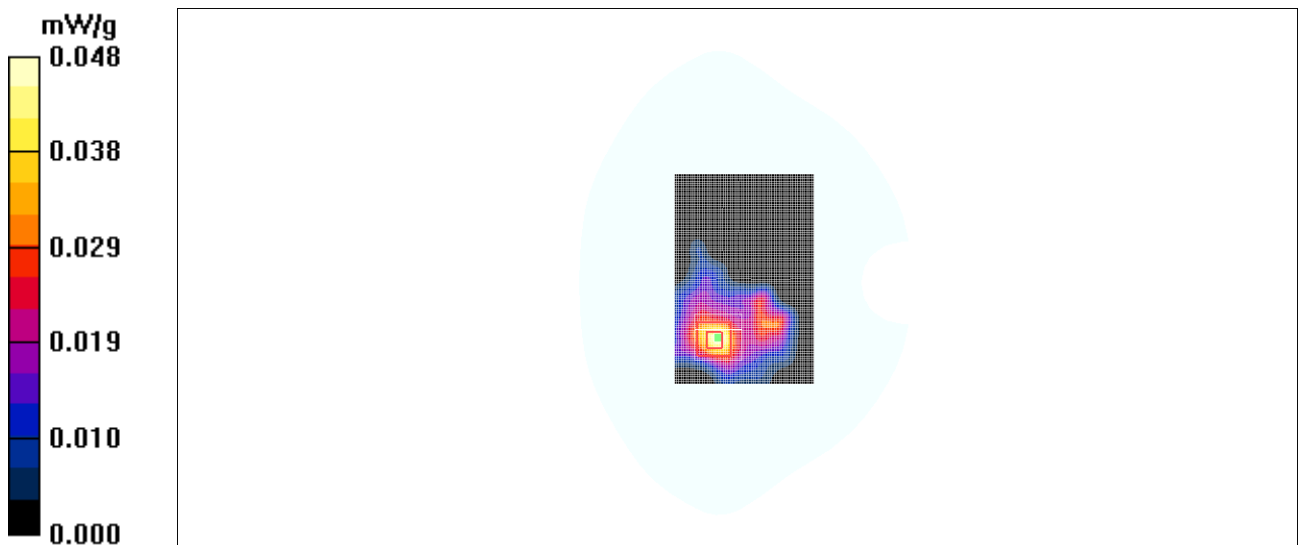
Fig.182 802.11g 36Mbps CH11
