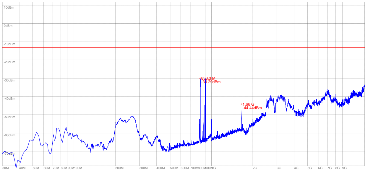
(Plot N.1: WCDMA 850MHz Channel = 4175, Test Antenna Horizontal)
