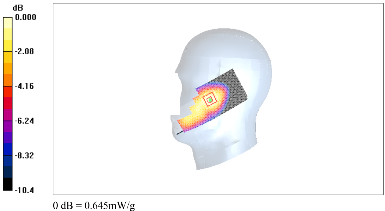
Fig. 7 850 MHz CH251
