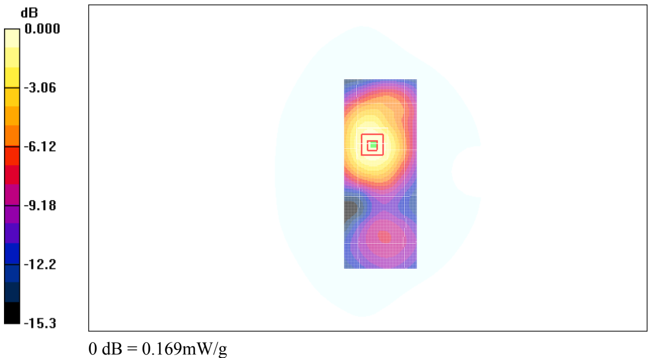
Fig. 32 1900 MHz CH810
