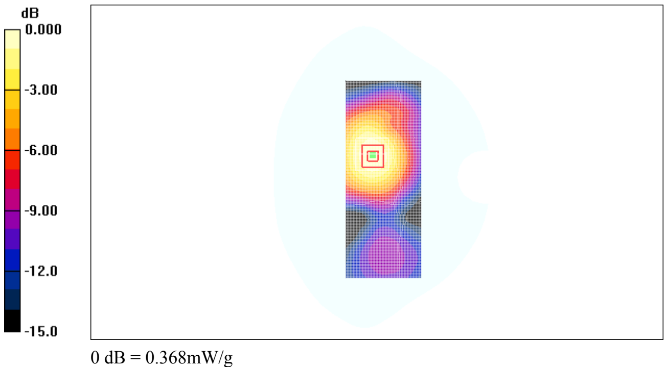
Fig. 29-1 1900 MHz CH810
