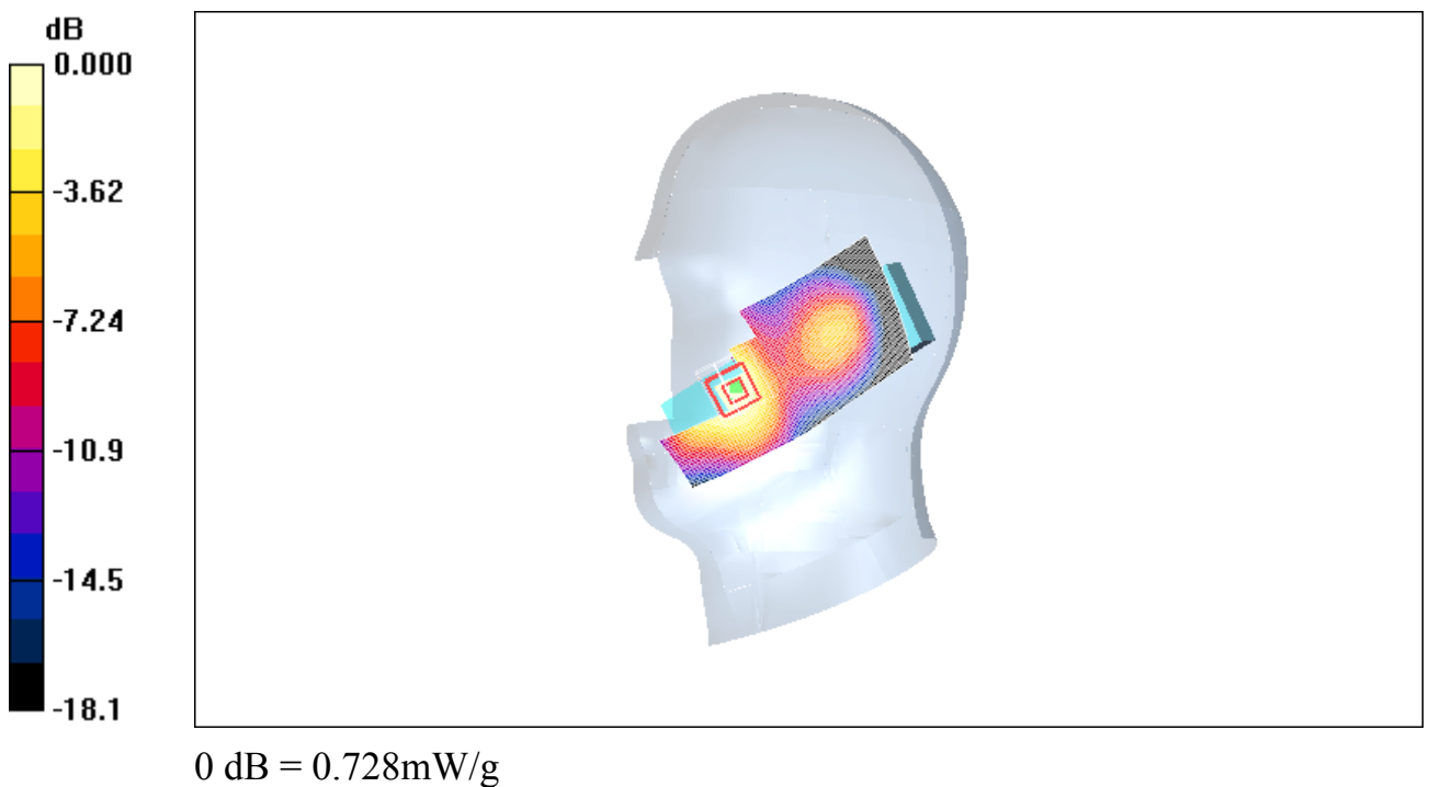
Fig. 24 1900 MHz CH661
