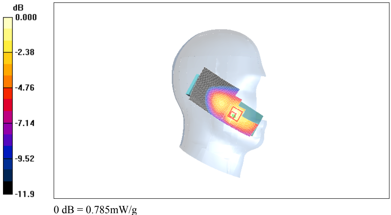
Fig. 1 850MHz CH251
