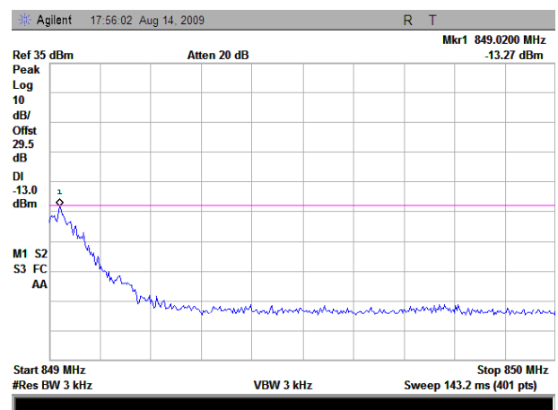
(Plot B1: GSM 850MHz_Channel = 251)
