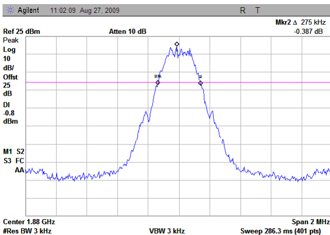
(Plot E2: EDGE 1900MHz Channel = 661)
