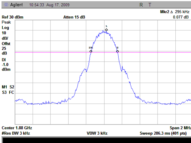
(Plot E1: GSM 1900MHz Channel = 661)
