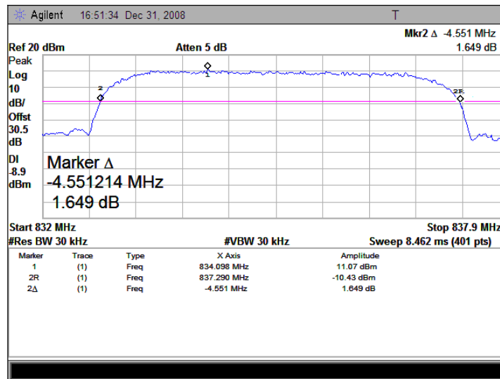
(Plot A: WCDMA 850MHz Channel = 4175)
