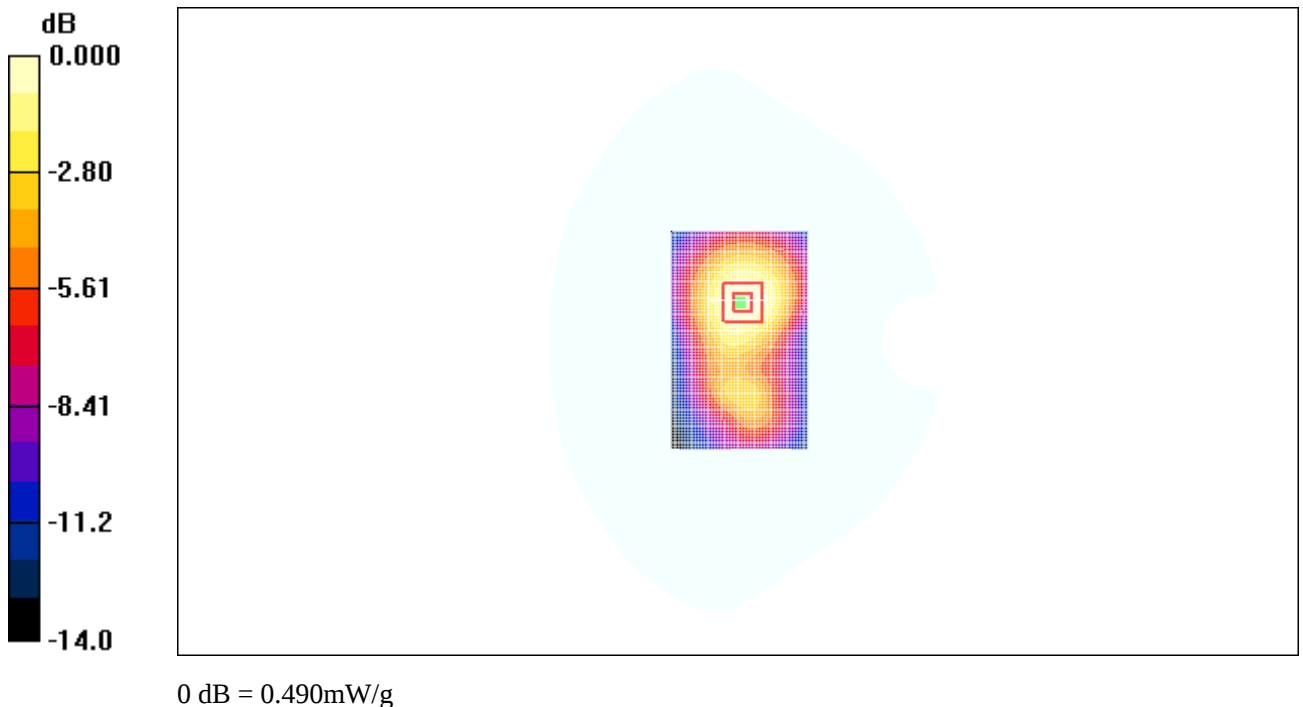
Fig. 65 1900 MHz CH810
