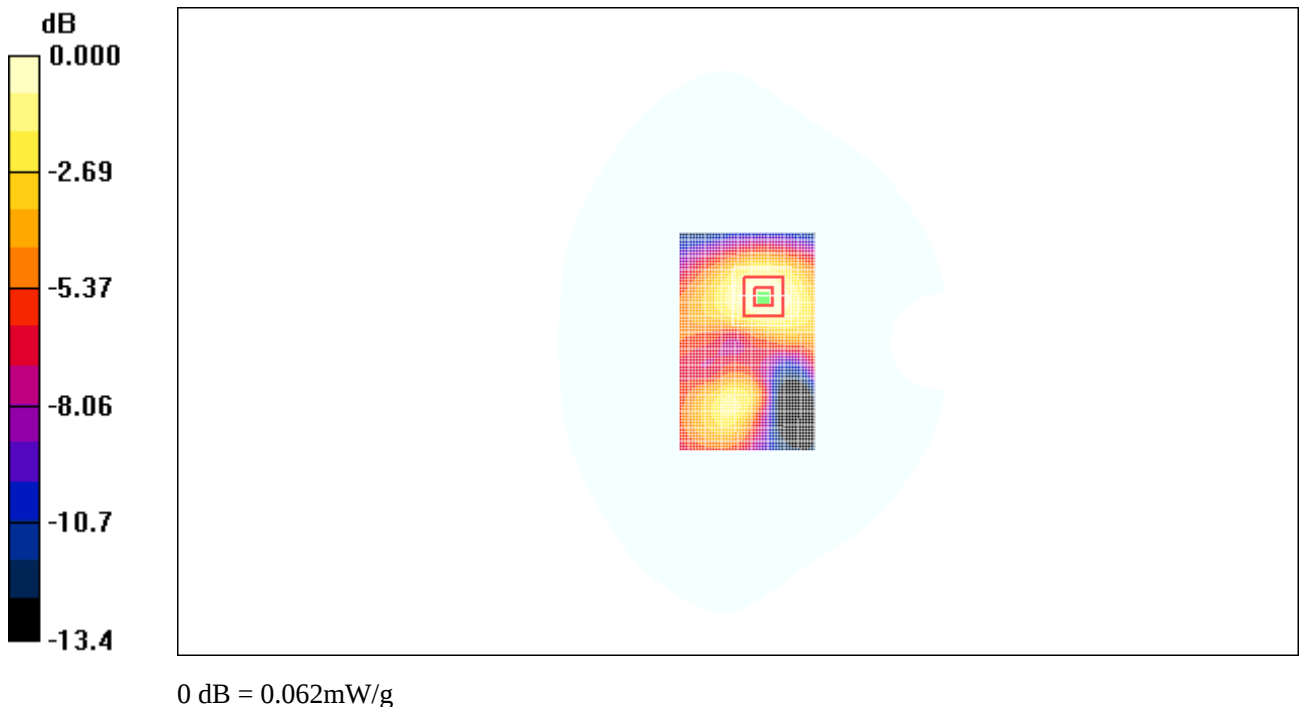
Fig. 71 1900 MHz CH810
