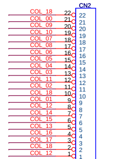
FPC Conn 22pin , 1.0mm 180度
