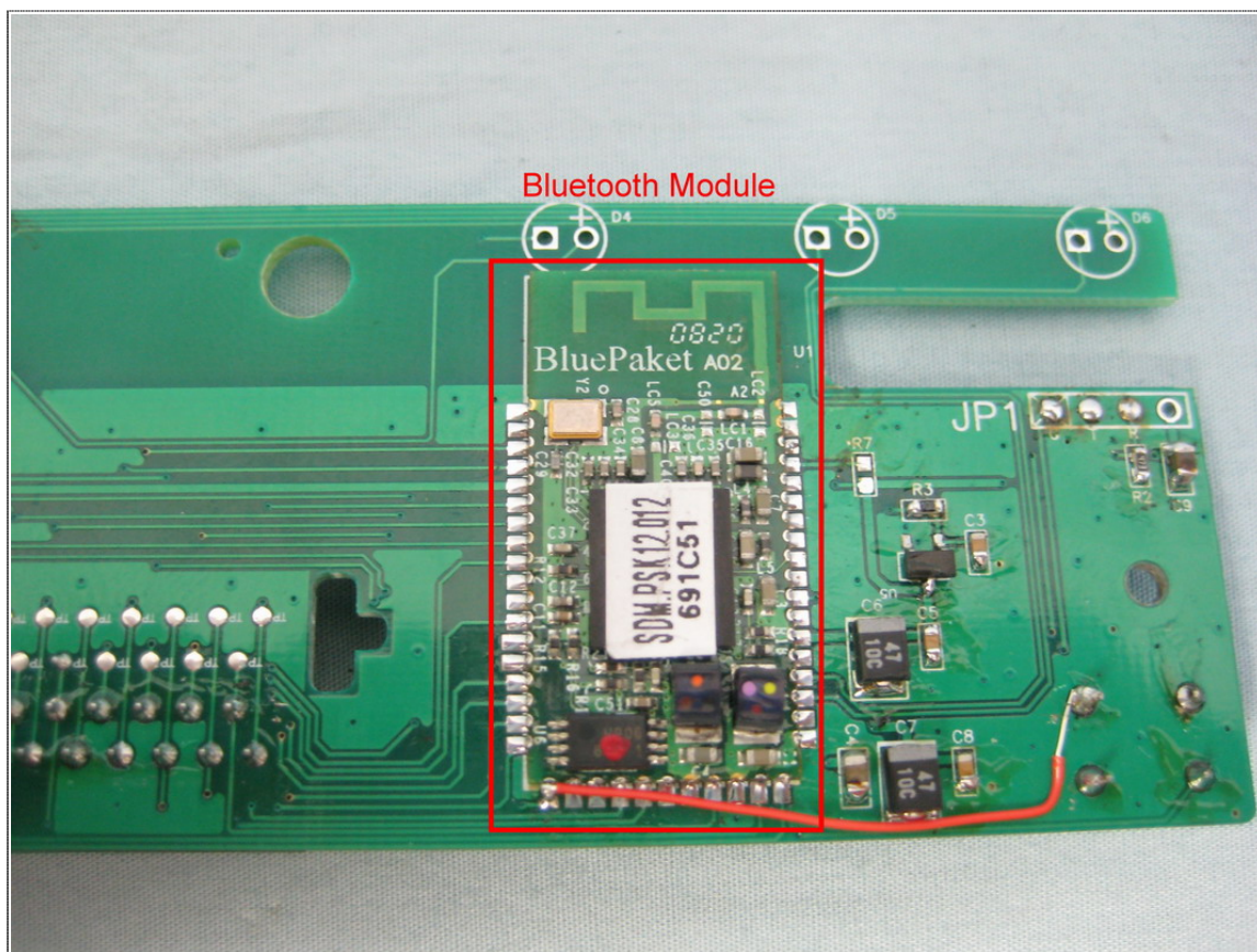
Bluetooth Module
