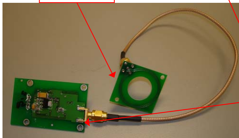
RFID Antenna
