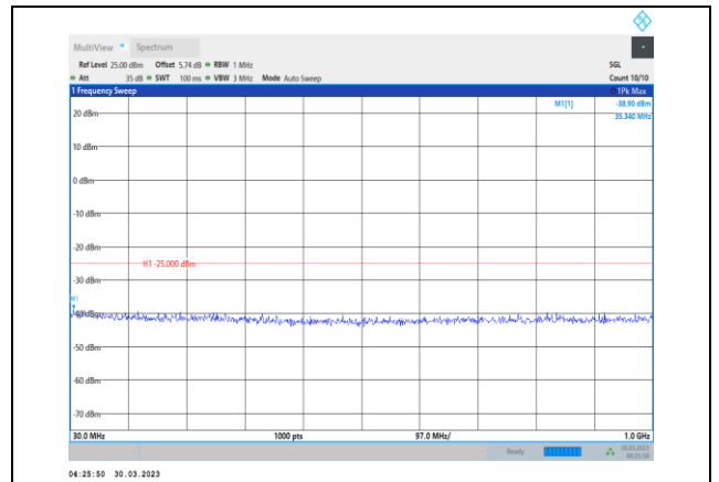
Band41-10MHz-QPSK-39700-1RB#0- Range1:30~1000MHz
