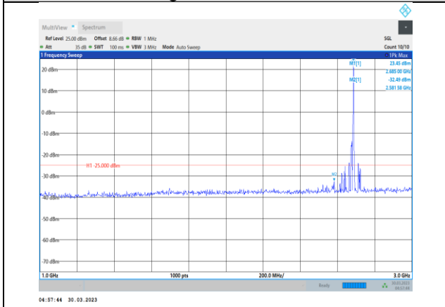
Band41-5MHz-QPSK-41565-1RB#0- Range2:1000~3000MHz
