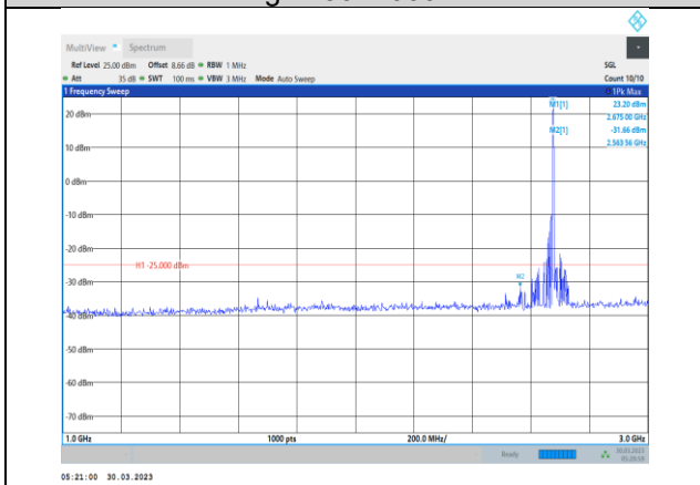
Band41-15MHz-QPSK-41515-1RB#0- Range2:1000~3000MHz
