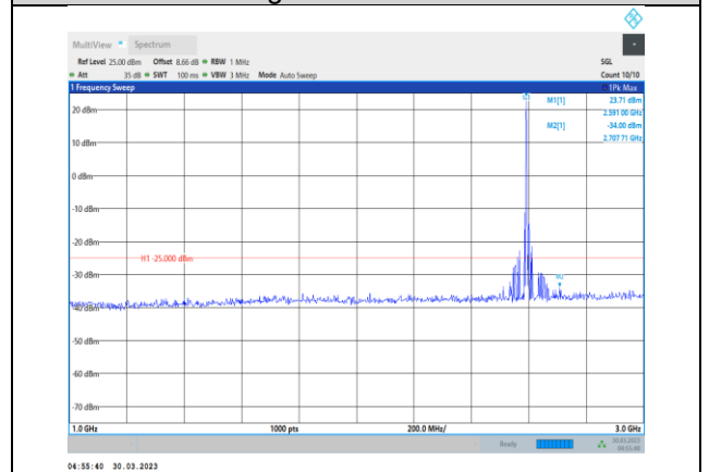
Band41-5MHz-QPSK-40620-1RB#0- Range2:1000~3000MHz
