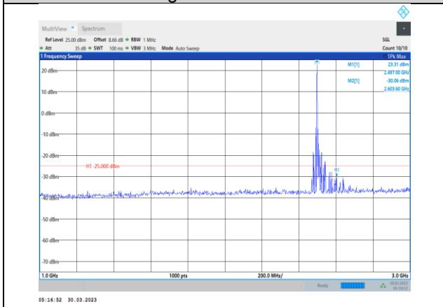
Band41-15MHz-QPSK-39725-1RB#0- Range2:1000~3000MHz
