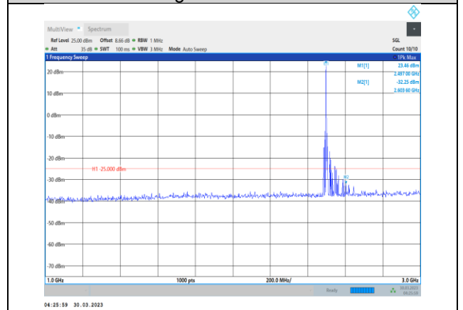
Band41-10MHz-QPSK-39700-1RB#0- Range2:1000~3000MHz
