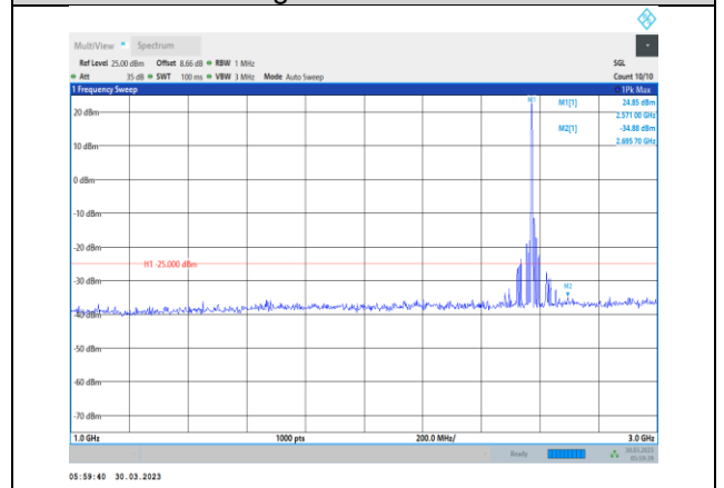
Band38-20MHz-64QAM-37850-1RB#0- Range2:1000~3000MHz
