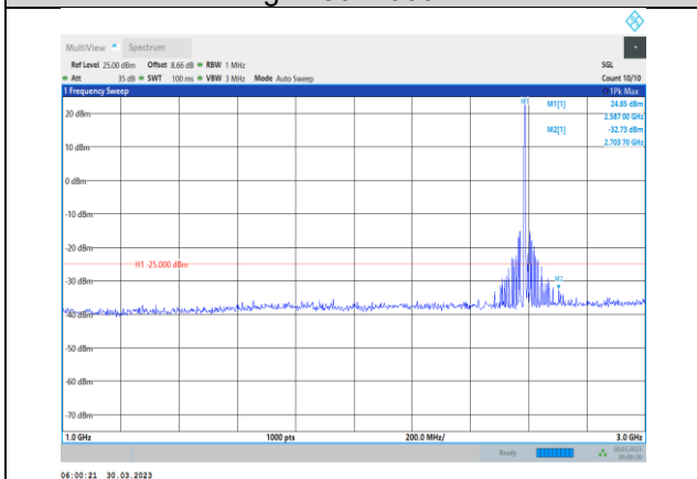
Band38-20MHz-QPSK-38000-1RB#0- Range2:1000~3000MHz
