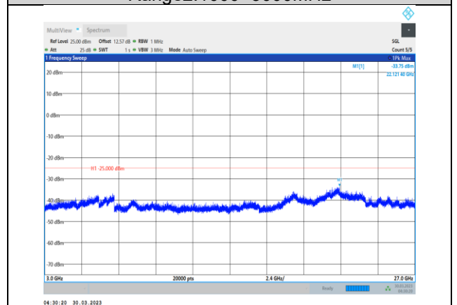
Band41-10MHz-QPSK-41540-1RB#0- Range3:3000~27000MHz
