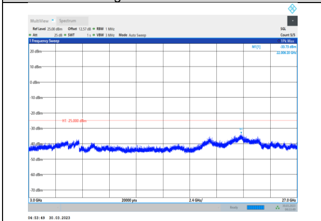
Band41-5MHz-QPSK-39675-1RB#0- Range3:3000~27000MHz
