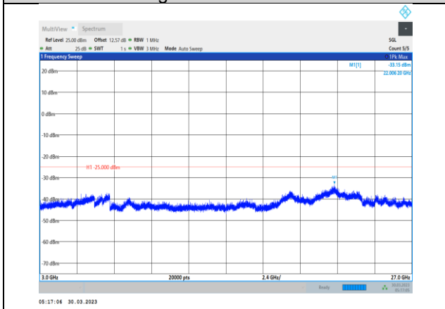
Band41-15MHz-QPSK-39725-1RB#0- Range3:3000~27000MHz
