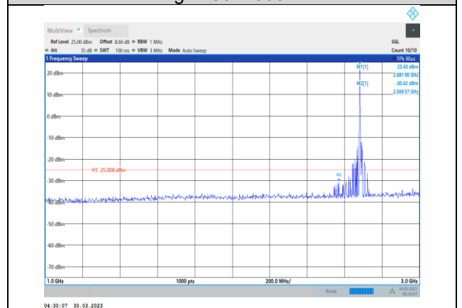
Band41-10MHz-QPSK-41540-1RB#0- Range2:1000~3000MHz
