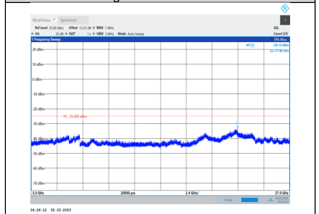
Band41-10MHz-QPSK-39700-1RB#0- Range3:3000~27000MHz
