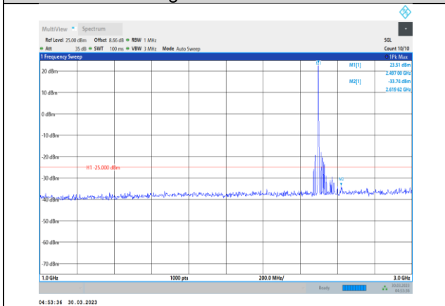
Band41-5MHz-QPSK-39675-1RB#0- Range2:1000~3000MHz
