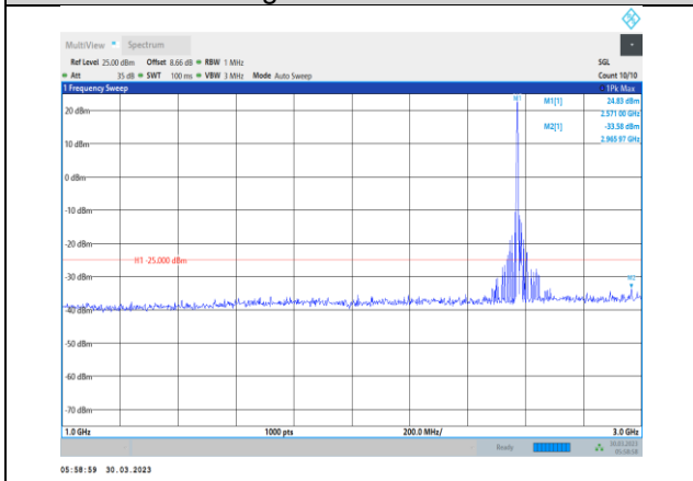
Band38-20MHz-16QAM-37850-1RB#0- Range2:1000~3000MHz
