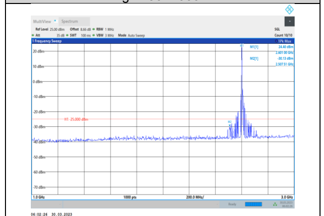
Band38-20MHz-QPSK-38150-1RB#0- Range2:1000~3000MHz
