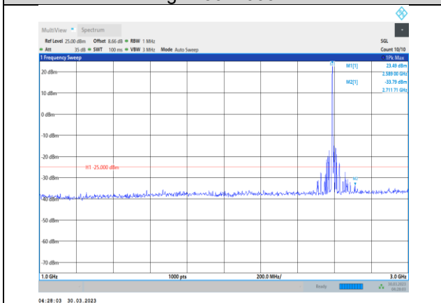
Band41-10MHz-QPSK-40620-1RB#0- Range2:1000~3000MHz
