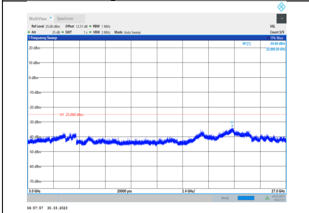
Band41-5MHz-QPSK-41565-1RB#0- Range3:3000~27000MHz
