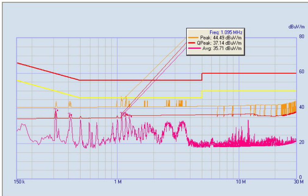
(Plot D: N Phase)
