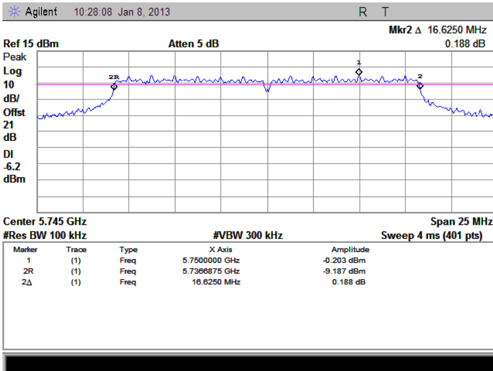
(Plot A: Channel 149: 5745MHz @ 802.11a)
