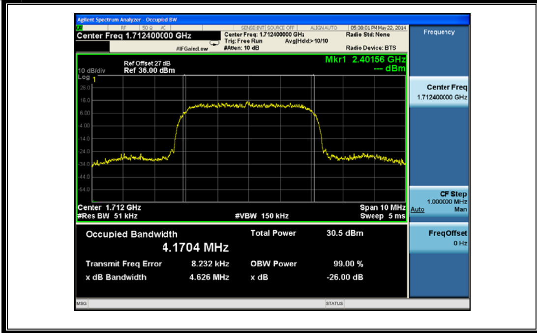
(Plot Q1: HSUPA 1700MHz Channel = 1312)
