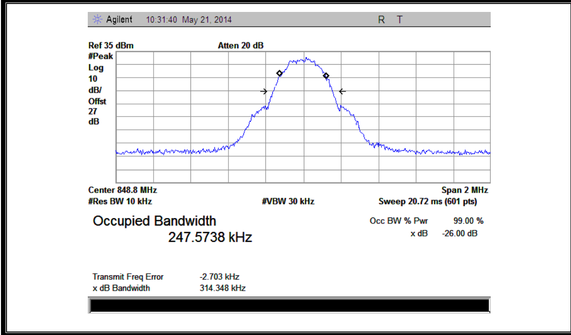
(PlotY1: GPRS850MHz Channel = 251)
