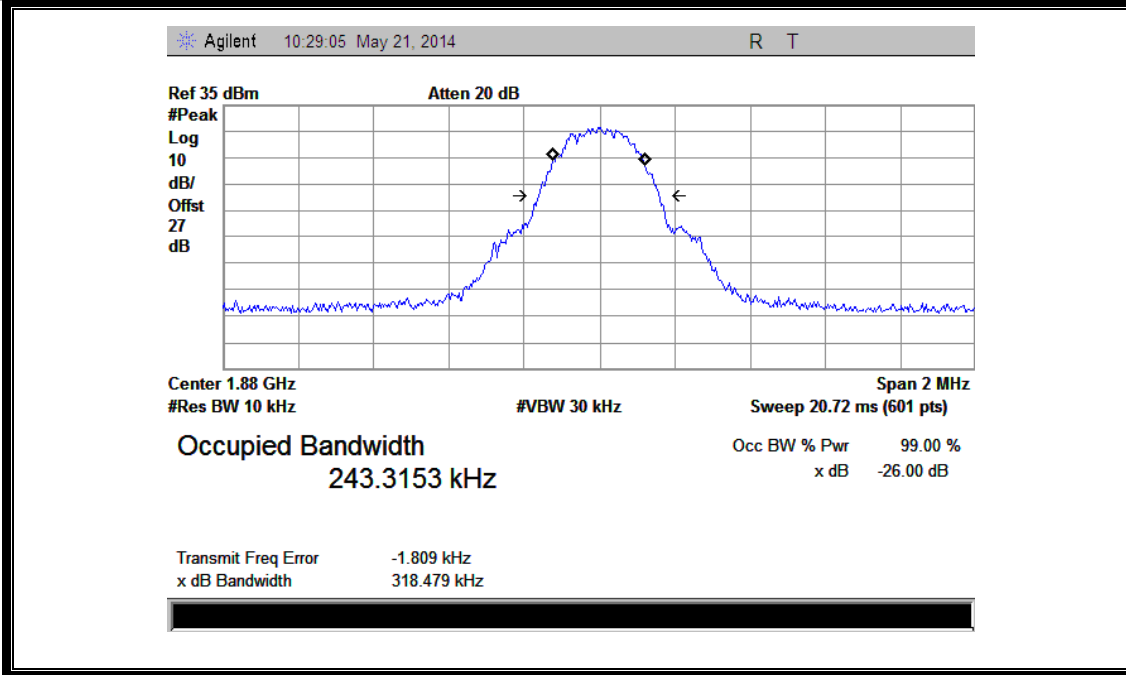
(Plot A2:GPRS 1900MHz Channel = 661)
