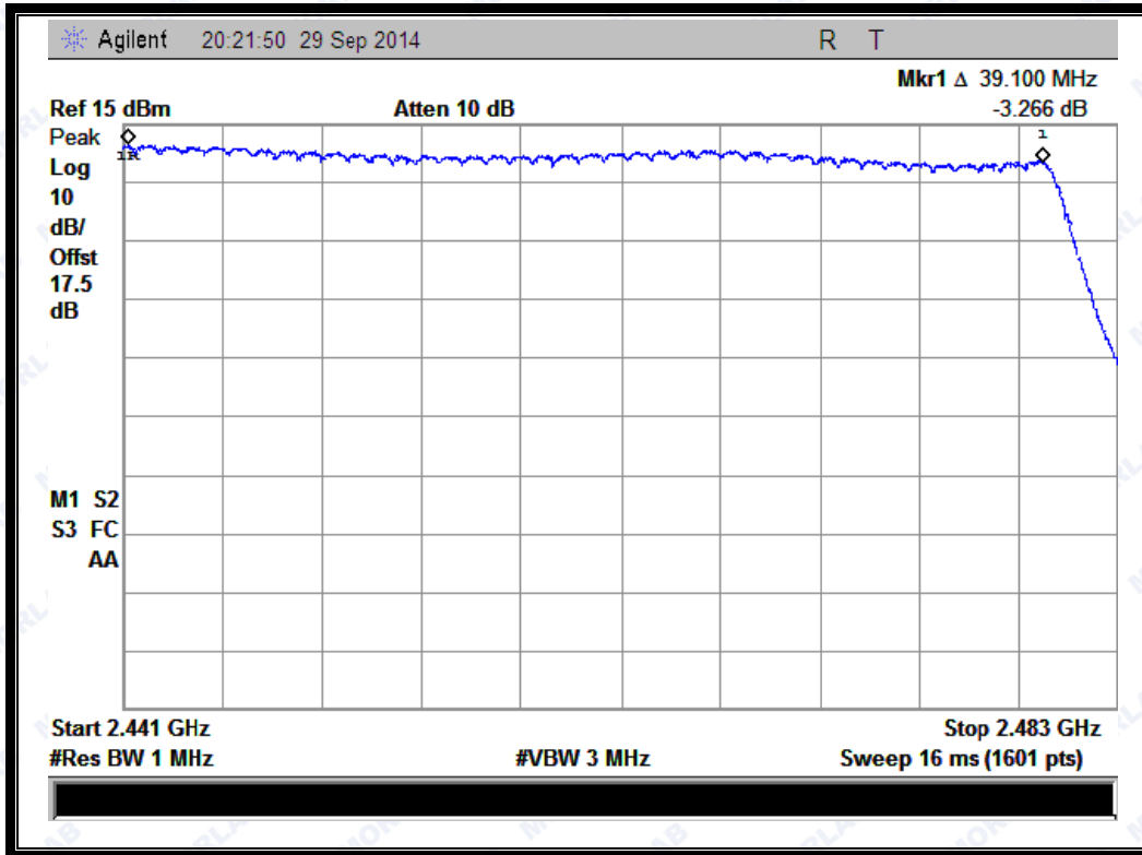
(Plot B: □/4-DQPSK)
