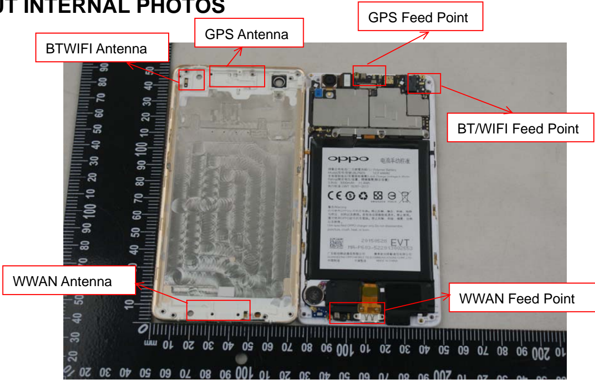
EUT Photo 1
