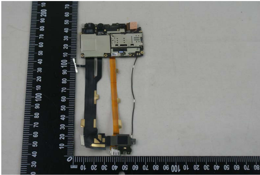
EUT Photo 5
