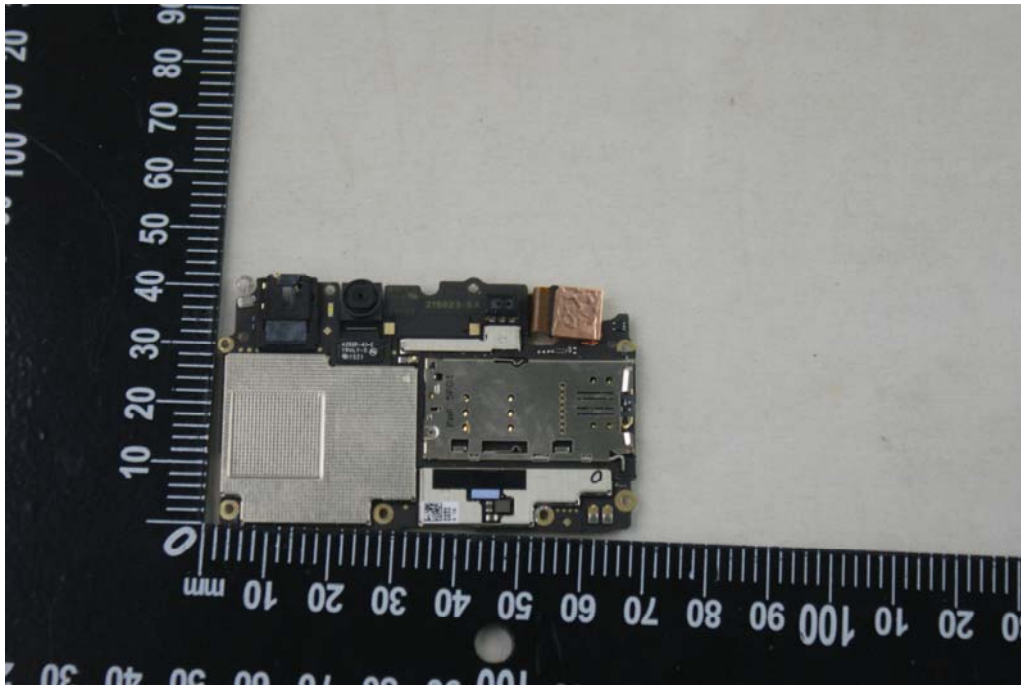
EUT Photo 7
