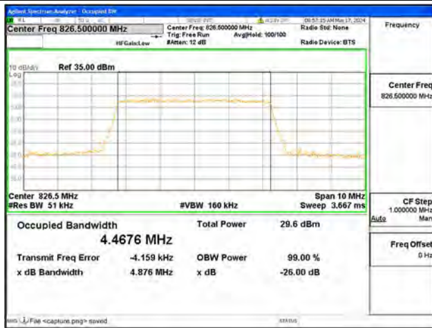
B18 part22 / 5MHz / QPSK/ Low CH
