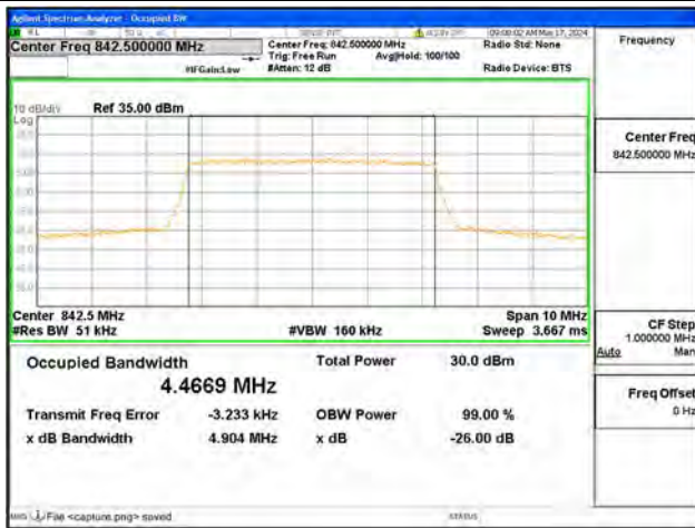
B19 / 5MHz / QPSK/ High CH
