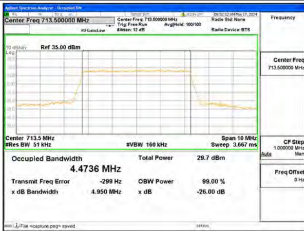
B17 / 5MHz / QPSK/ High CH
