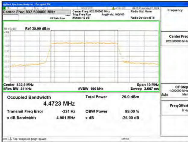
B19 / 5MHz / QPSK/ Low CH
