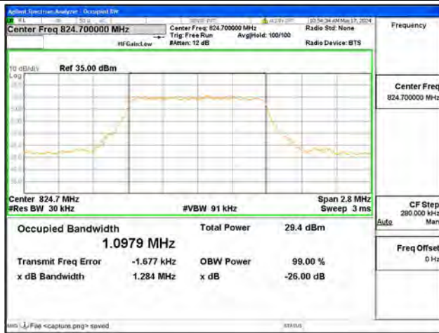
B26 Part22 / 1.4MHz / QPSK/ Low CH
