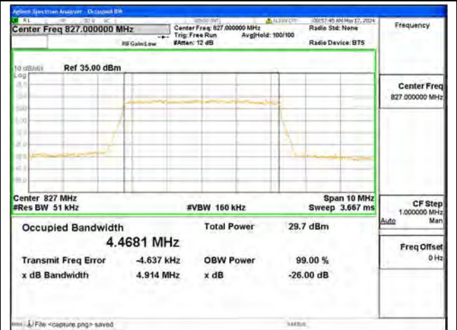
B18 part22 / 5MHz / QPSK/ Mid CH
