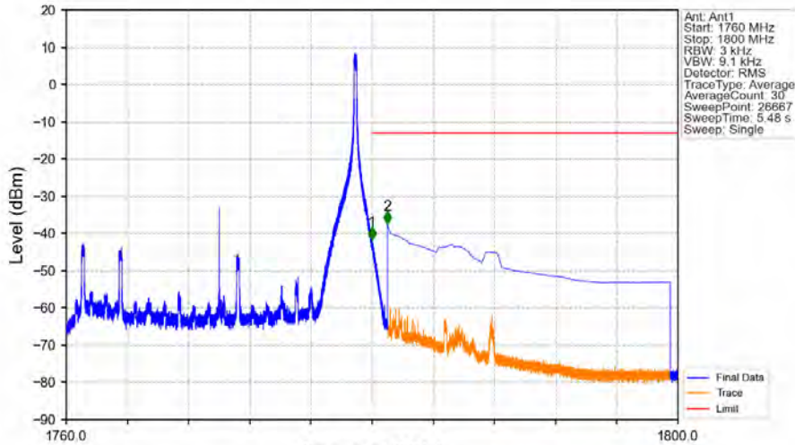
Band66_20MHz_QPSK_HCH_1770MHz_RB_1_99_NTNV
