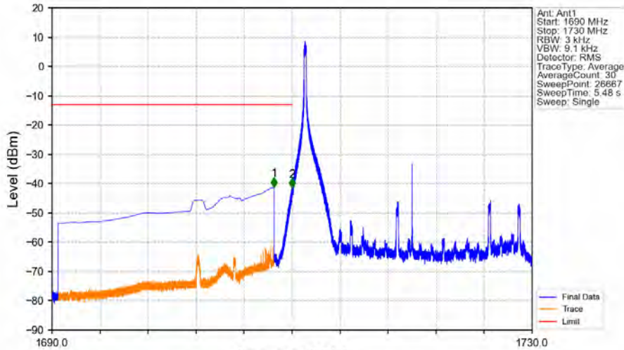
Band66_20MHz_16QAM_LCH_1720MHz_RB_1_0_NTNV
