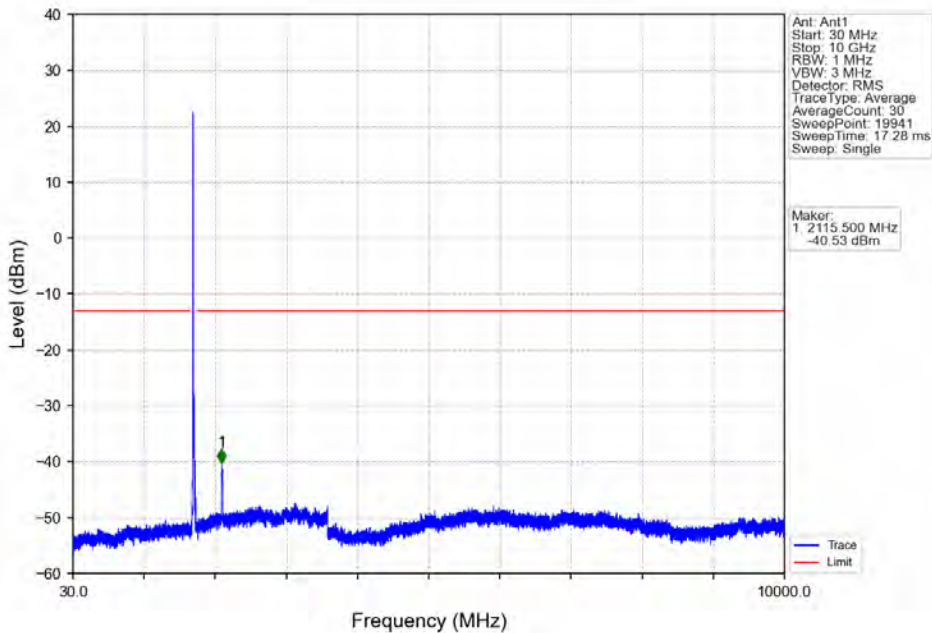
Band66_20MHz_QPSK_LCH_1720MHz_RB_1_0_NTNV
