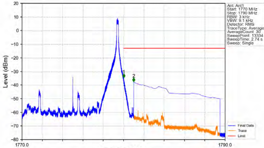
Band66_10MHz_QPSK_HCH_1775MHz_RB_1_49_NTNV
