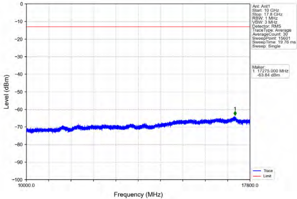
Band66_20MHz_QPSK_MCH_1745MHz_RB_1_0_NTNV
