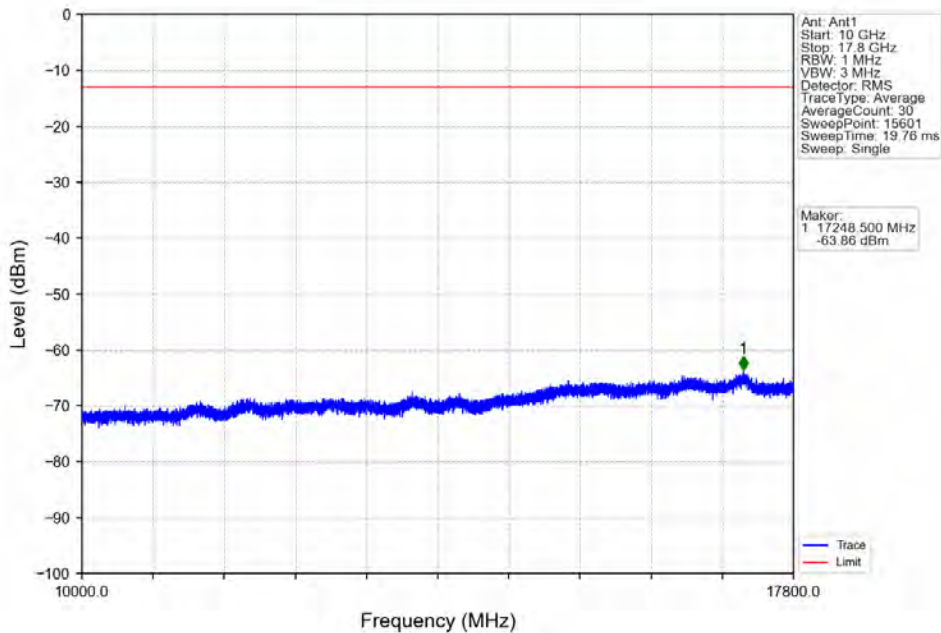
Band66_20MHz_QPSK_HCH_1770MHz_RB_1_0_NTNV
