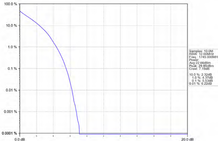
Band66_10MHz QPSK MCH_1745MHz_RB_50_0_NTNV
