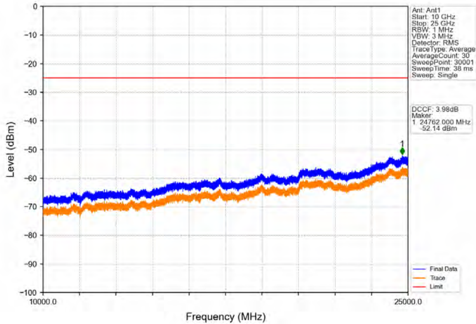
Band41_20MHz_QPSK_MCH_2593MHz_RB_1_0_NTNV
