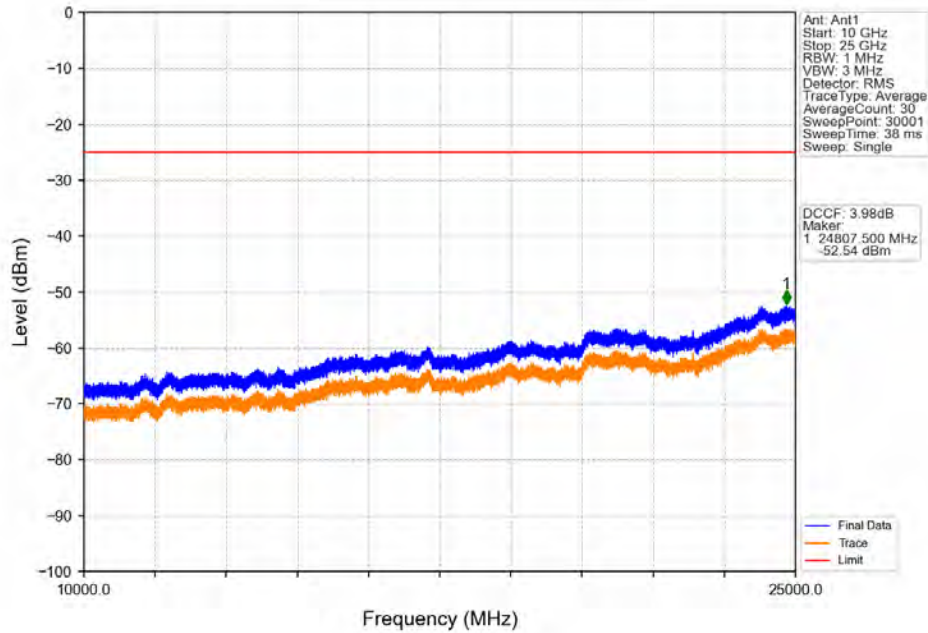
Band41_15MHz_QPSK_MCH_2593MHz_RB_1_0_NTNV
