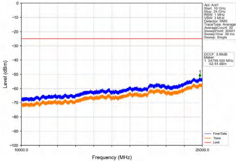
Band41_20MHz_QPSK_HCH_2680MHz_RB_1_0_NTNV
