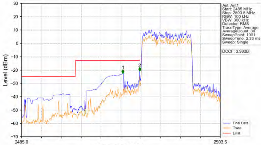
Band41_5MHz_QPSK_LCH_2498.5MHz_RB_25_0_NTNV
