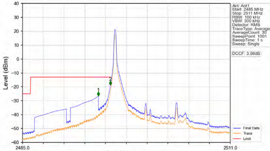
Band41_10MHz_16QAM_LCH_2501MHz_RB_1_0_NTNV
