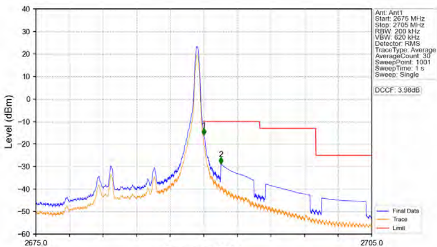
Band41_10MHz_QPSK_HCH_2685MHz_RB_1_49_NTNV
