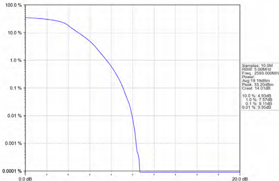
Band41_5MHz_QPSK_MCH_2593MHz_RB_25_0_NTNV
