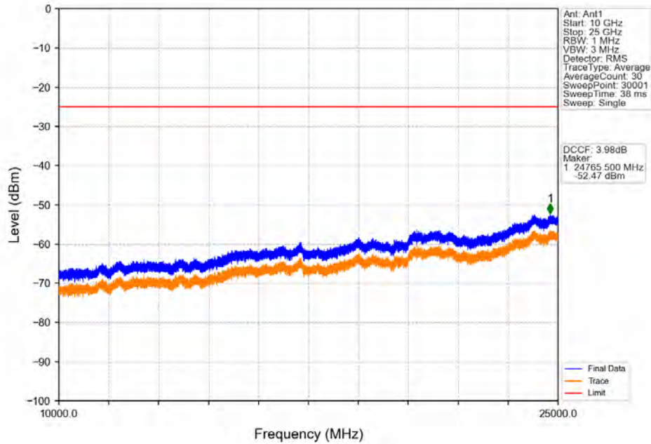
Band41_10MHz_QPSK_MCH_2593MHz_RB_1_0_NTNV
