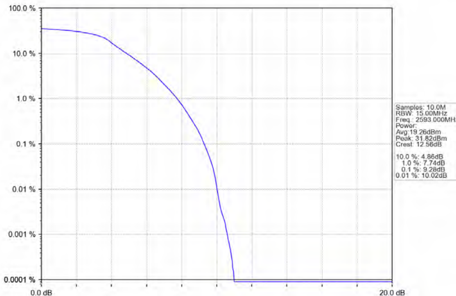
Band41_15MHz_QPSK_MCH_2593MHz_RB_75_0_NTNV
