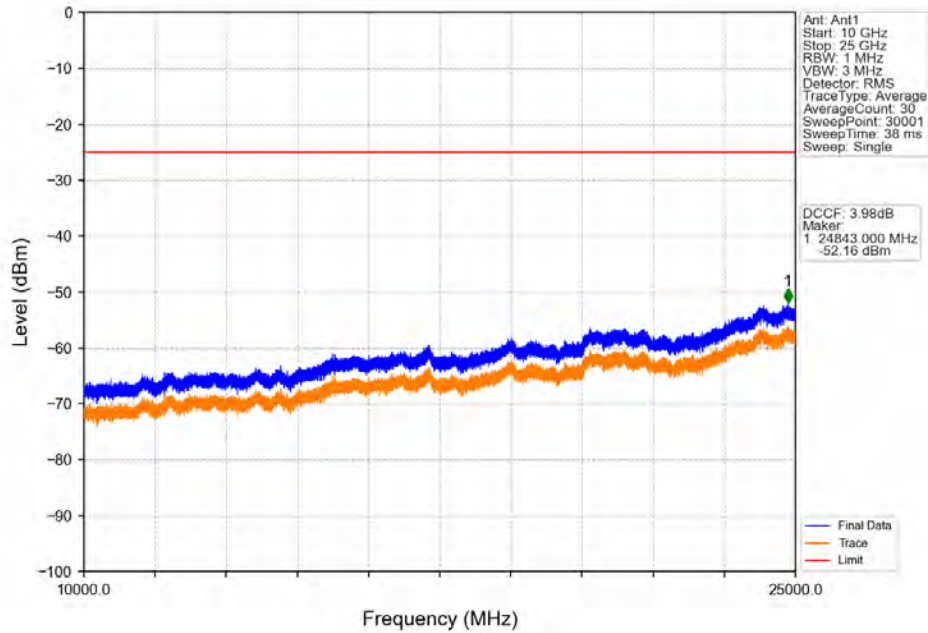
Band41_10MHz_16QAM_MCH_2593MHz_RB_1_0_NTNV
