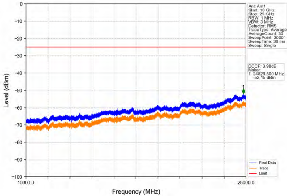
Band41_5MHz_QPSK_MCH_2593MHz_RB_1_0_NTNV
