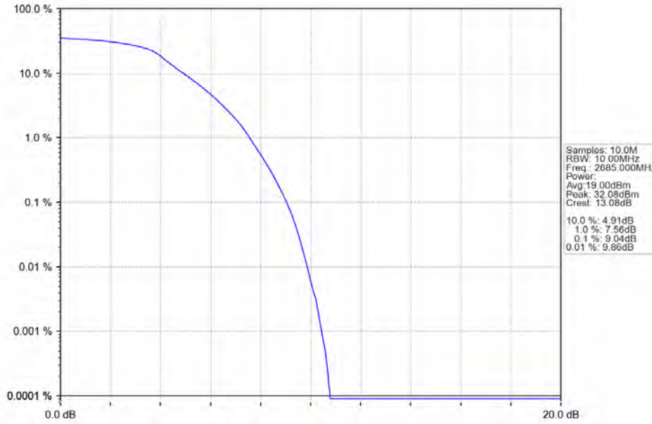
Band41_10MHz_QPSK_HCH_2685MHz_RB_50_0_NTNV
