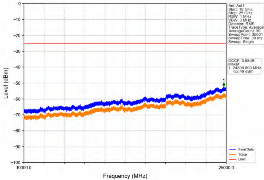
Band41_5MHz_QPSK_LCH_2498.5MHz_RB_1_0_NTNV
