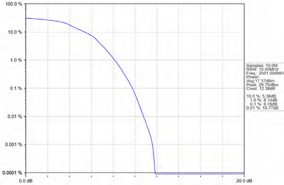
Band41_10MHz_16QAM_LCH_2501MHz_RB_50_0_NTNV
