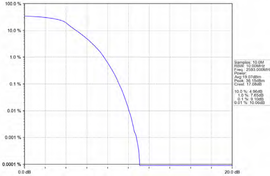
Band41_10MHz QPSK MCH_2593MHz_RB_50_0_NTNV
