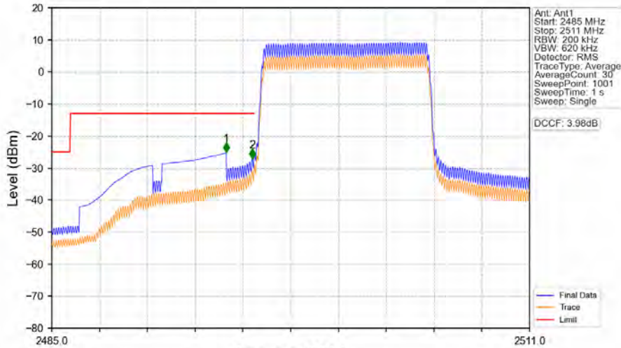
Band41_10MHz_QPSK_LCH_2501MHz_RB_50_0_NTNV
