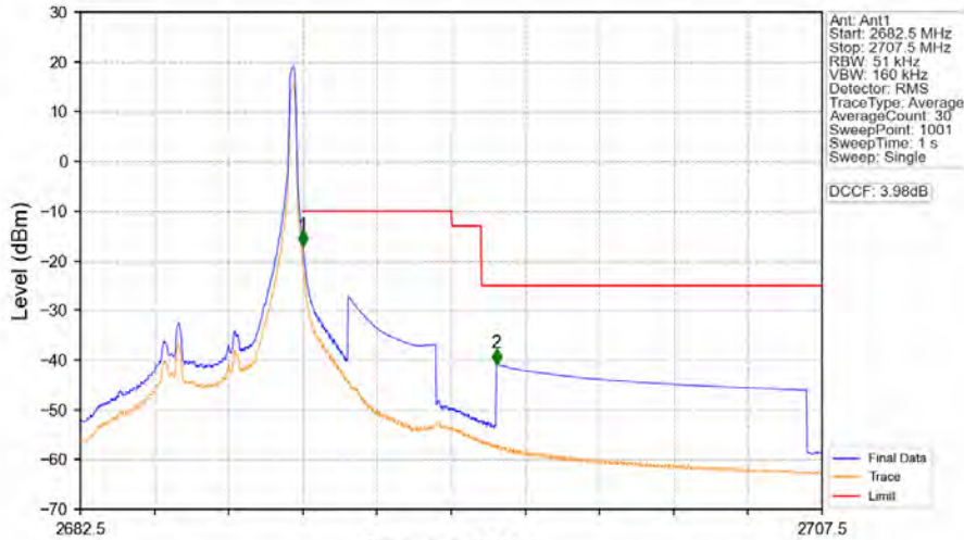
Band41_5MHz_QPSK_HCH_2687.5MHz_RB_1_24_NTNV
