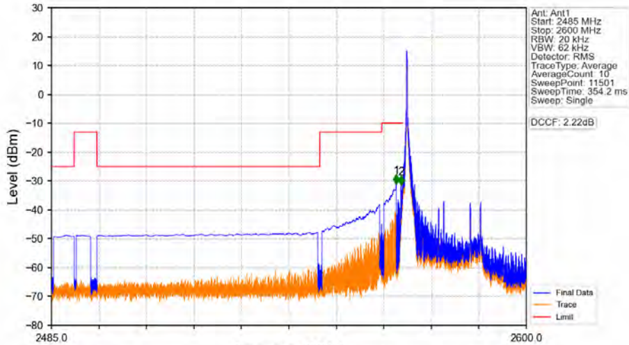
Band38_20MHz_16QAM_LCH_2580MHz_RB_1_0_NTNV
