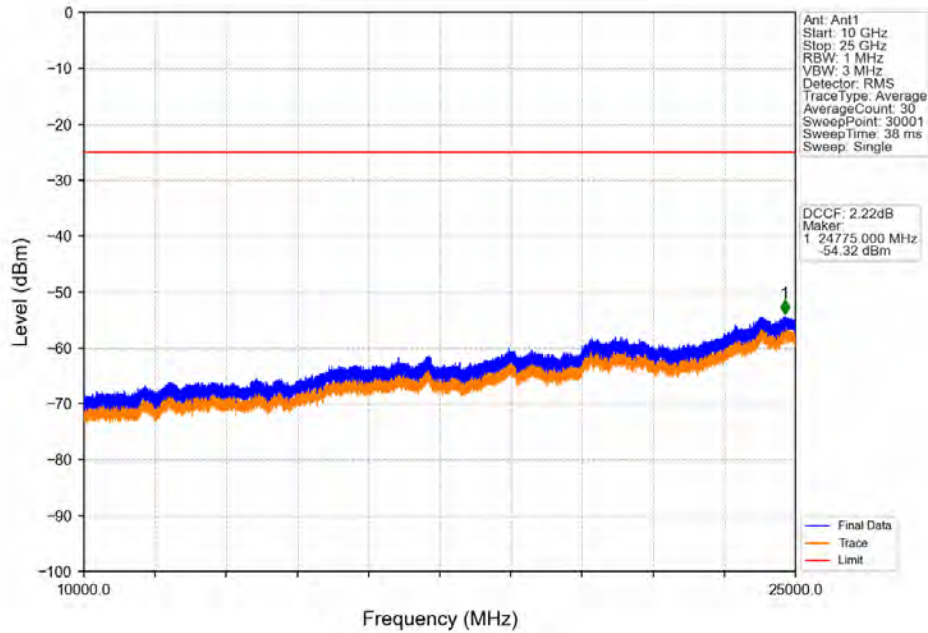
Band38_20MHz_QPSK_MCH_2595MHz_RB_1_0_NTNV
