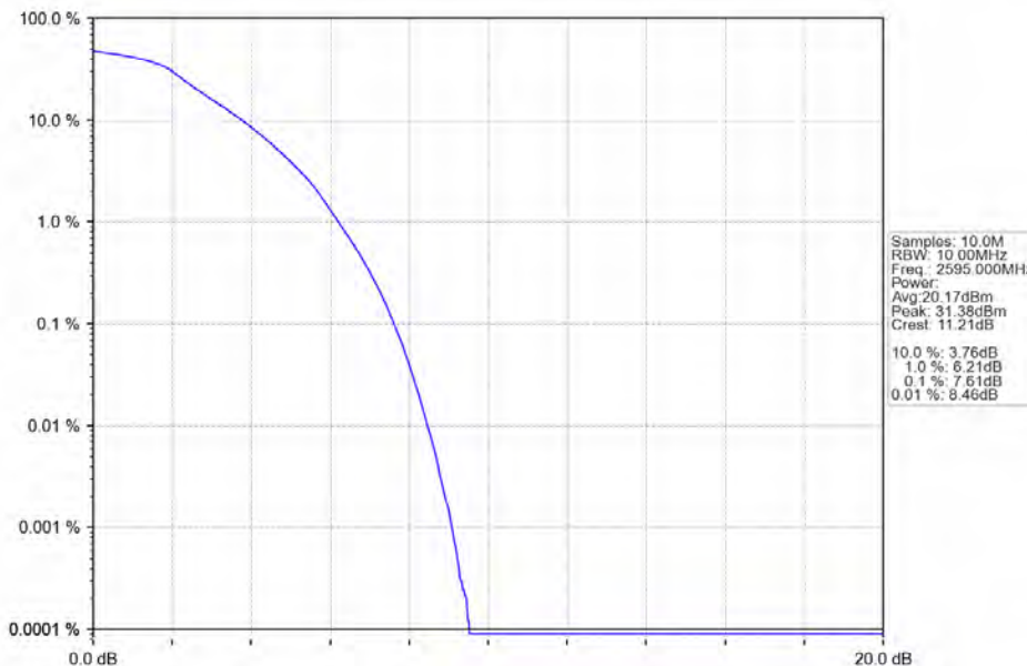
Band38_10MHz_QPSK_MCH_2595MHz_RB_50_0_NTNV
