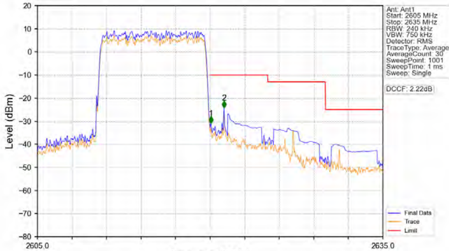
Band38_10MHz_QPSK_HCH_2615MHz_RB_50_0_NTNV
