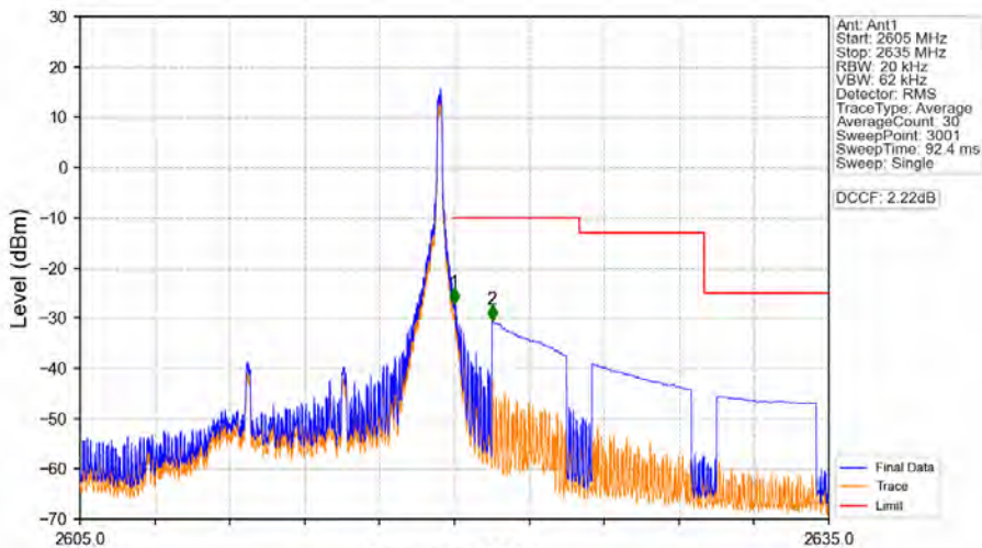
Band38_10MHz_QPSK_HCH_2615MHz_RB_1_49_NTNV
