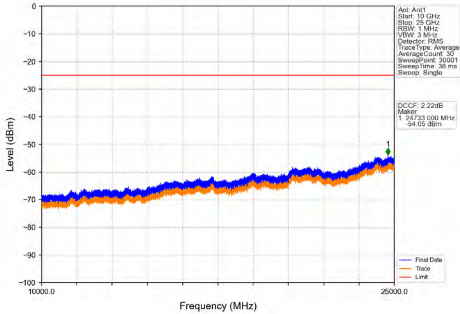
Band38_10MHz_QPSK_MCH_2595MHz_RB_1_0_NTNV
