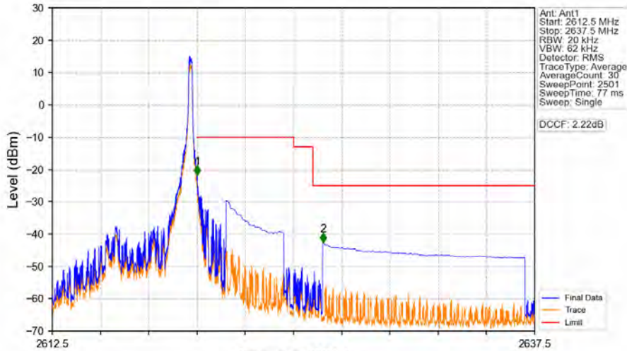
Band38_5MHz_QPSK_HCH_2617.5MHz_RB_1_24_NTNV
