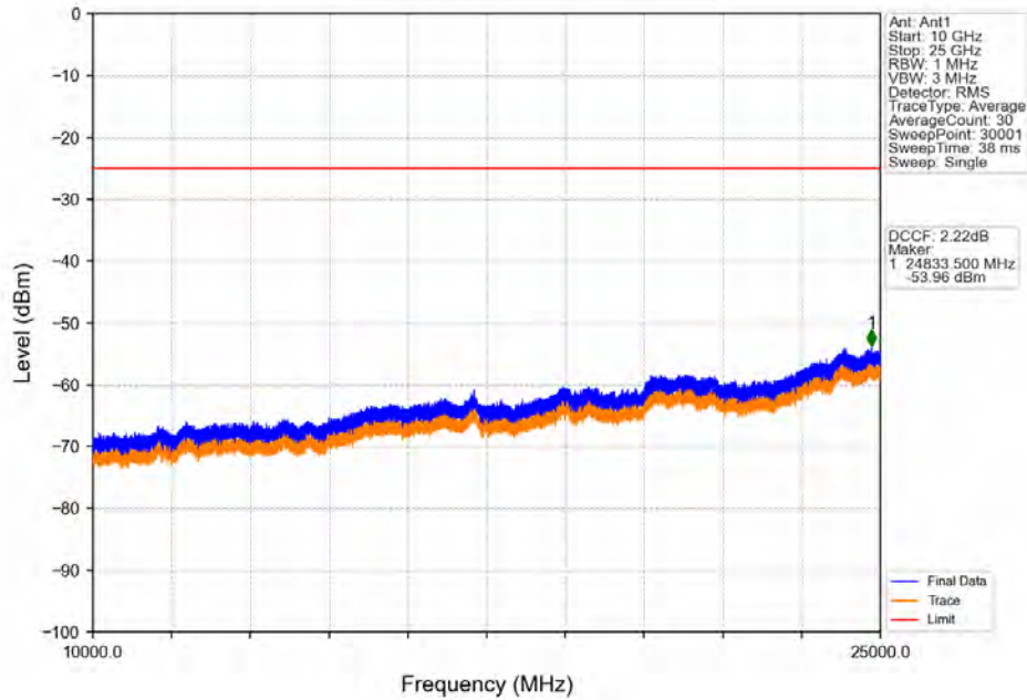
Band38_10MHz_QPSK_HCH_2615MHz_RB_1_0_NTNV
