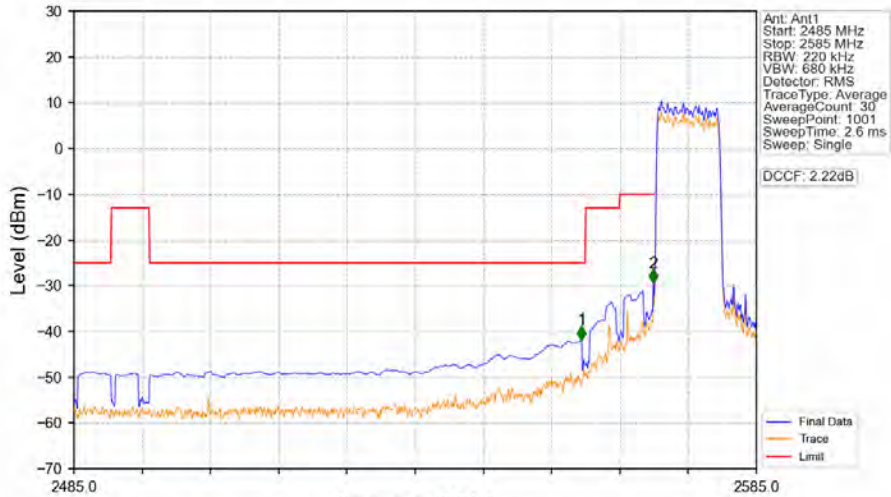
Band38_10MHz_QPSK_LCH_2575MHz_RB_50_0_NTNV
