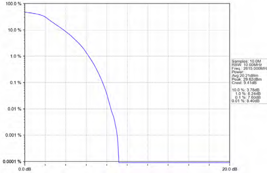
Band38_10MHz_QPSK_HCH_2615MHz_RB_50_0_NTNV
