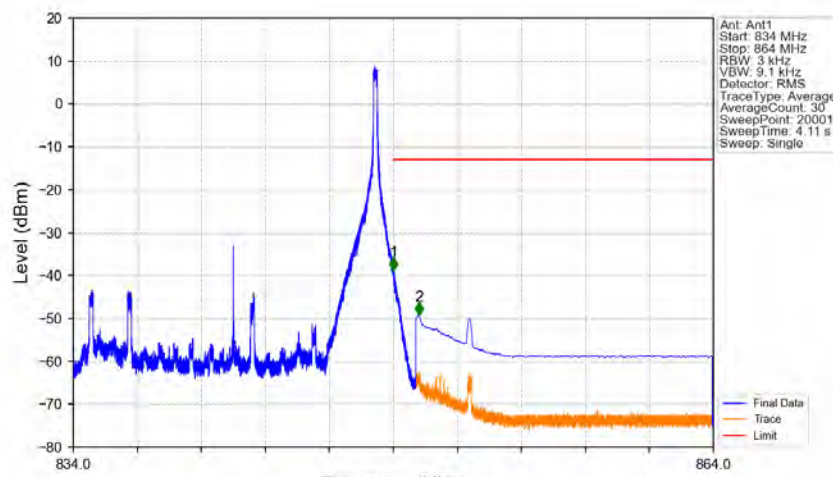
Band26b_15MHz_QPSK_HCH_841.5MHz_RB_1_74_NTNV
