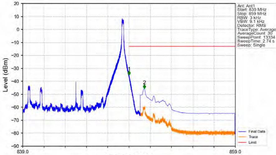
Band26b_10MHz_QPSK_HCH_844MHz_RB_1_49_NTNV
