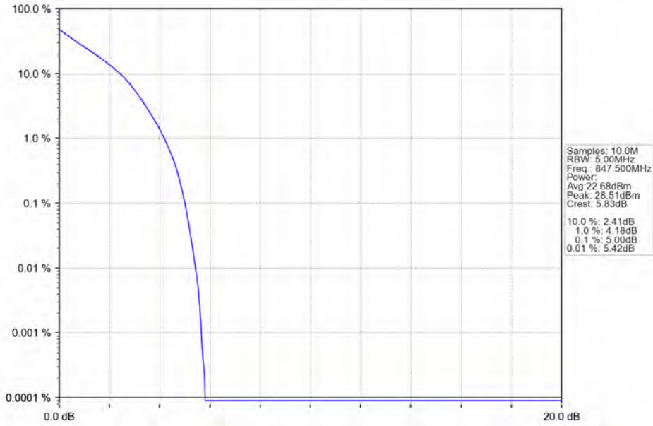
Band26b_3MHz_QPSK_HCH_847.5MHz_RB_15_0_NTNV
