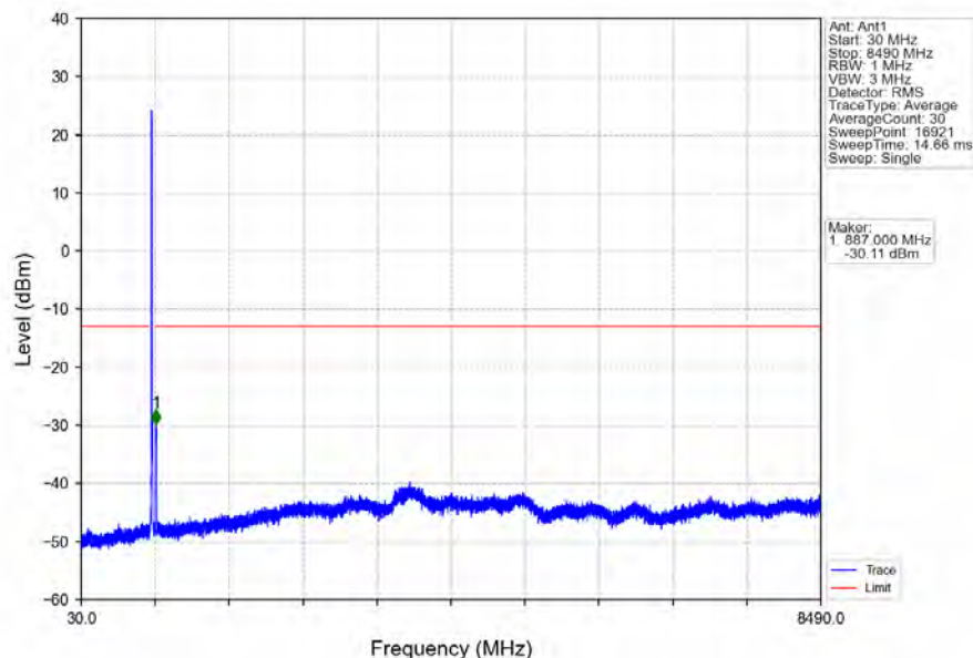
Band26b_15MHz_QPSK_HCH_841.5MHz_RB_1_74_NTNV
