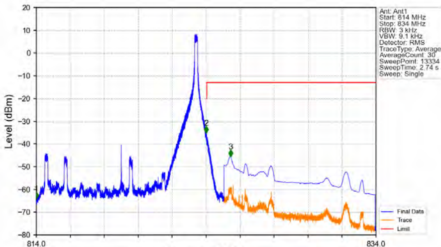
Band26a_10MHz_QPSK_HCH_819MHz_RB_1_49_NTNV
